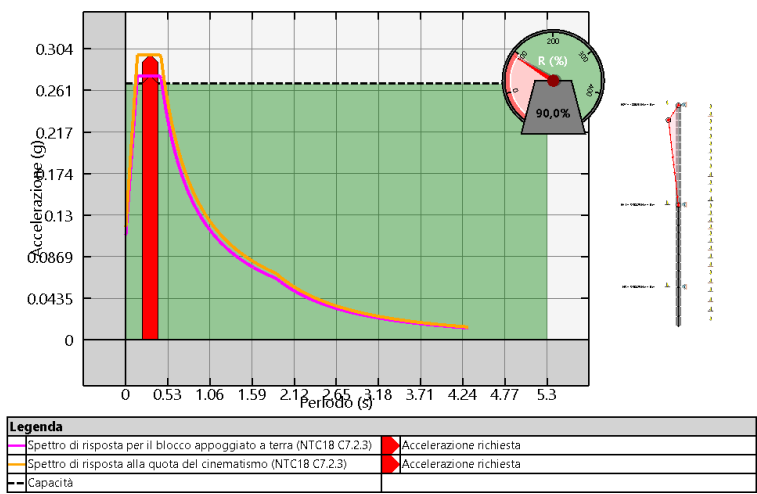
Cinematisimo più pericoloso allo SLD per: Fascia 21.1
