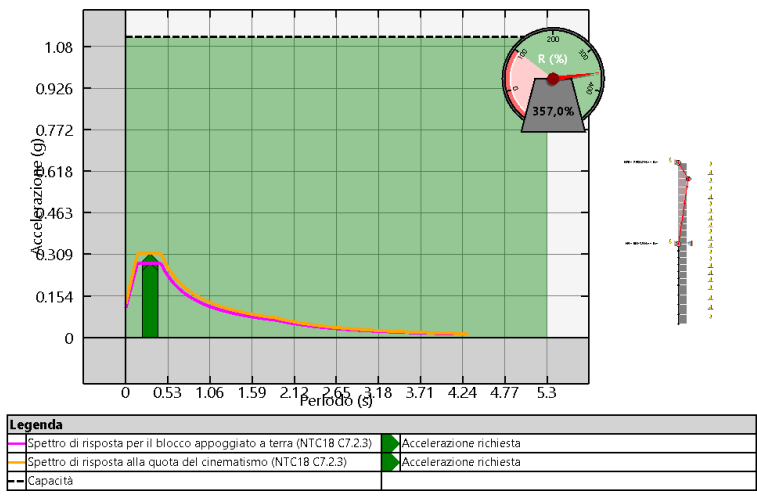
Cinematisimo più pericoloso allo SLD per: Fascia 11.1
