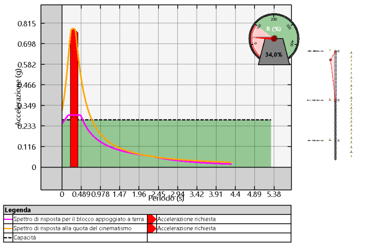
Cinematiso più pericoloso allo SLU per: Fascia 23.1
