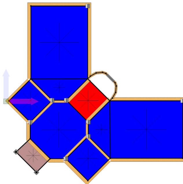
Pianta a quota 196 cm: carichi di area applicati ai solai
