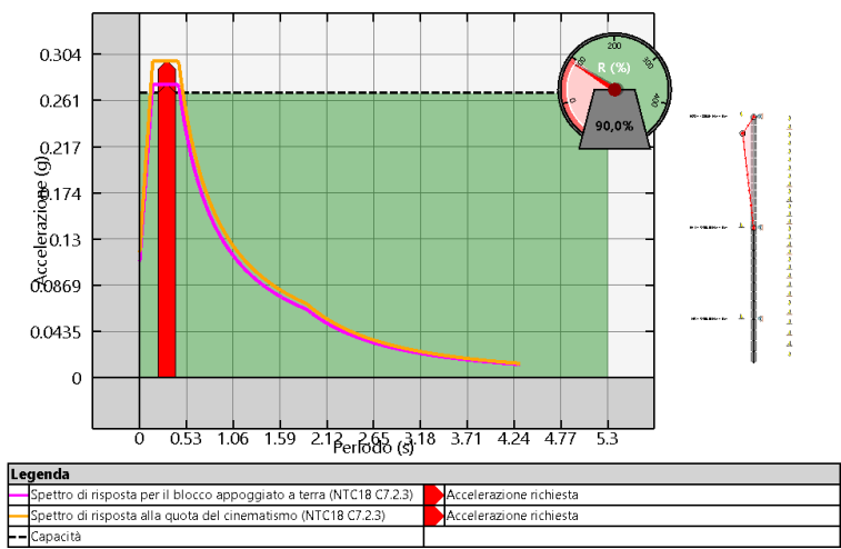
Cinematisimo più pericoloso allo SLD per: Fascia 27.1
