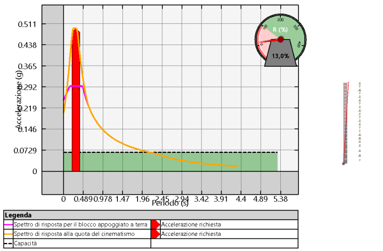
Cinematisimo più pericoloso allo SLU per: Fascia 16.1
