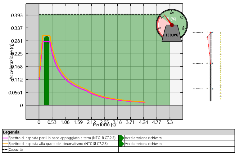
Cinematiso più pericoloso allo SLD per: Fascia 24.1
