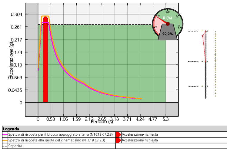
Cinematisimo più pericoloso allo SLD per: Fascia 25.1
