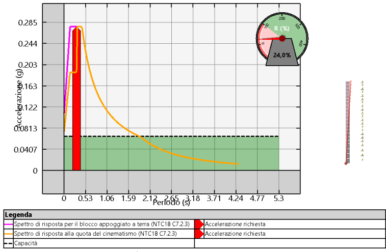
Cinematisimo più pericoloso allo SLD per: Fascia 16.1
