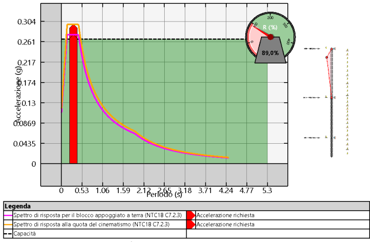
Cinematiso più pericoloso allo SLD per: Fascia 23.1
