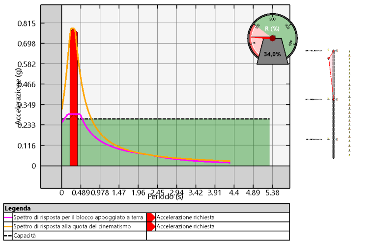
Cinematisimo più pericoloso allo SLU per: Fascia 26.1
