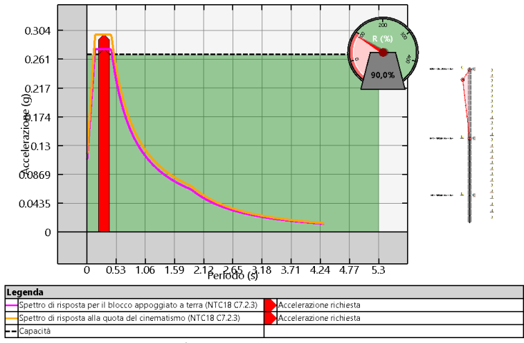
Cinematisimo più pericoloso allo SLD per: Fascia 26.1
