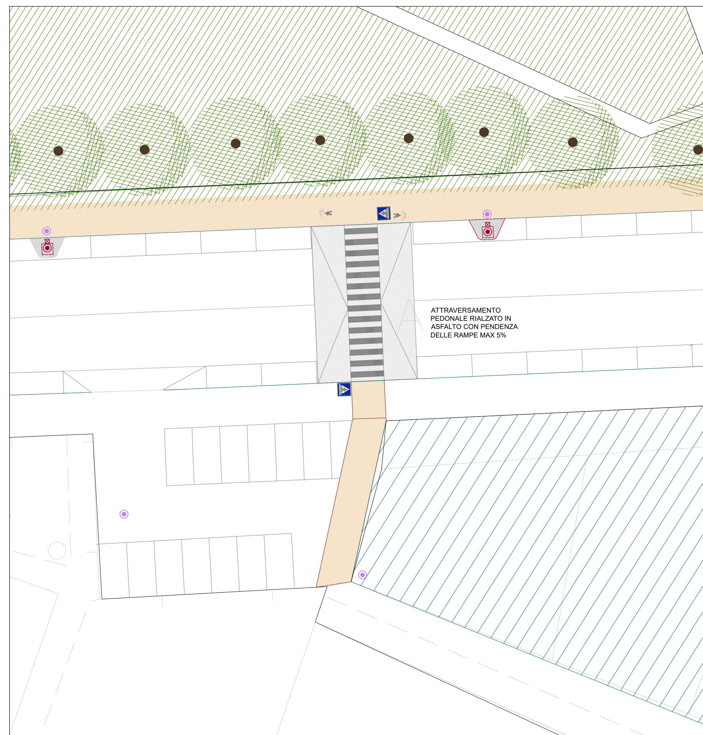
PARTICOLARE C - ATTRAVERSAMENTO RIALZATO SCALA 1:200
