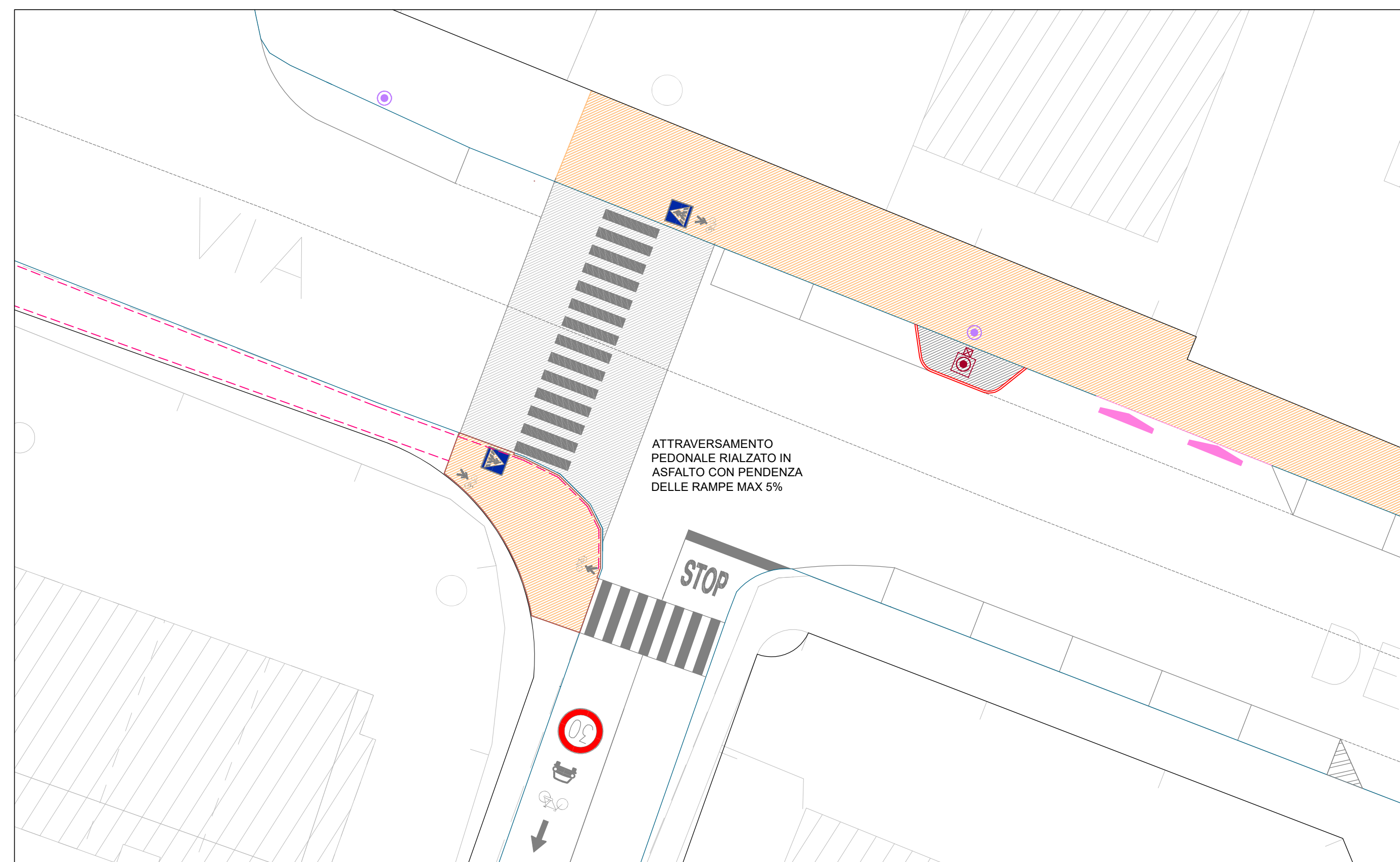
PARTICOLARE A - ATTRAVERSAMENTO RIALZATO SCALA 1:200
