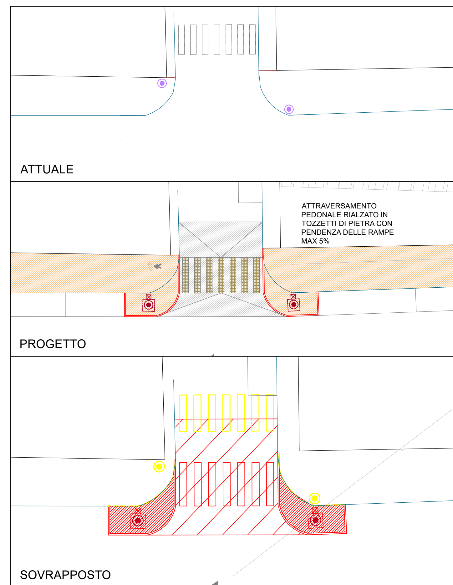
PARTICOLARE B - ATTRAVERSAMENTO RIALZATO SCALA 1:200
