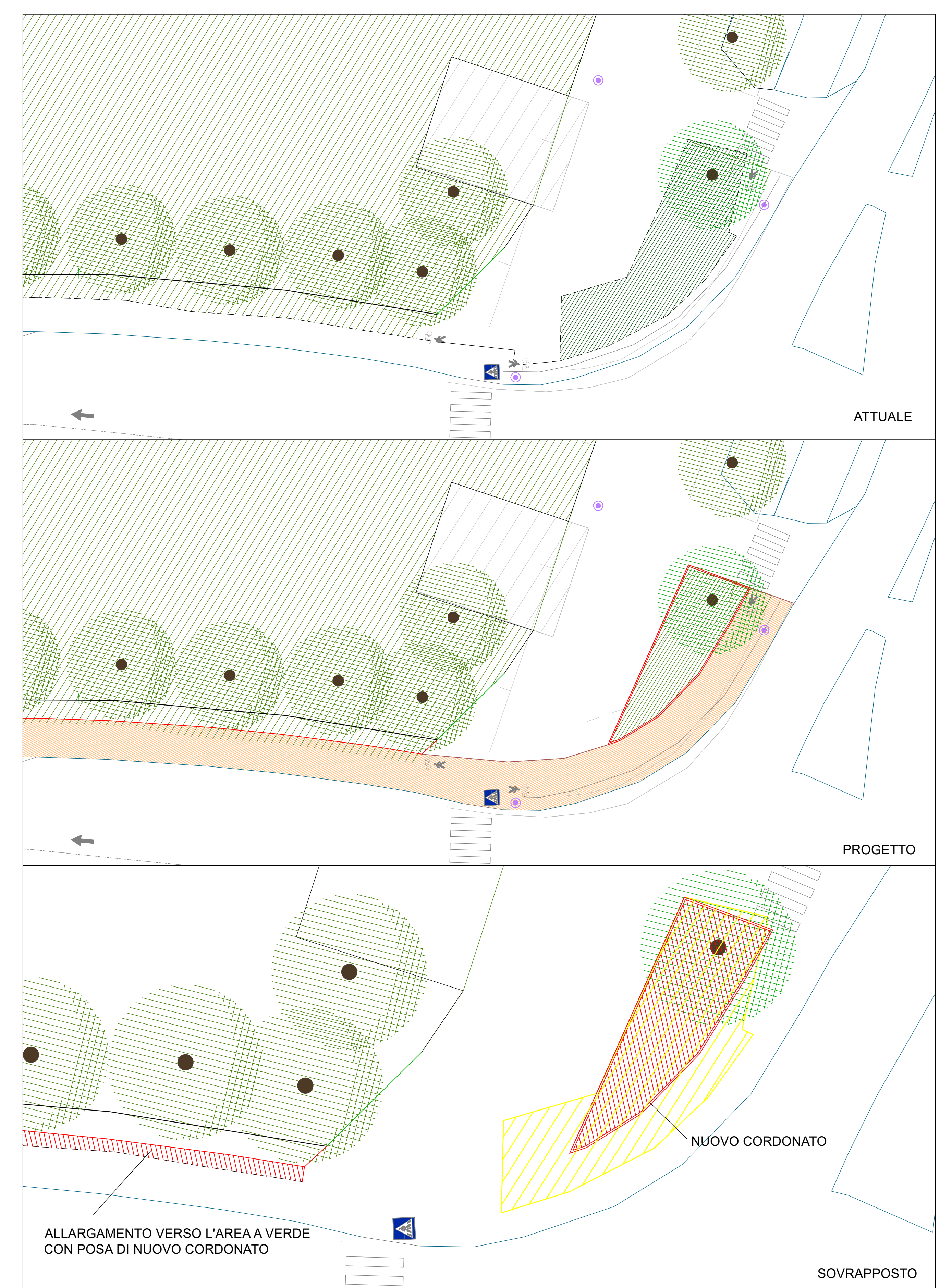
PARTICOLARE D - RACCORDO CON PISTA CICLABILE ESISTENTE SCALA 1:200
