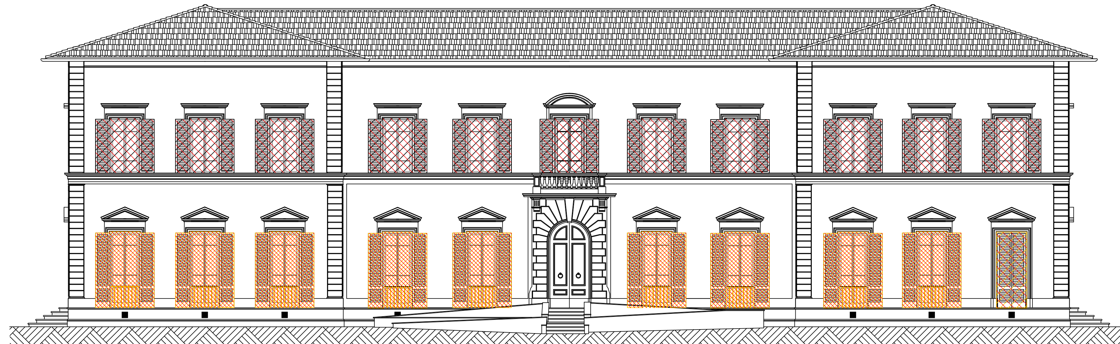
PROSPETTO FRONTALE
