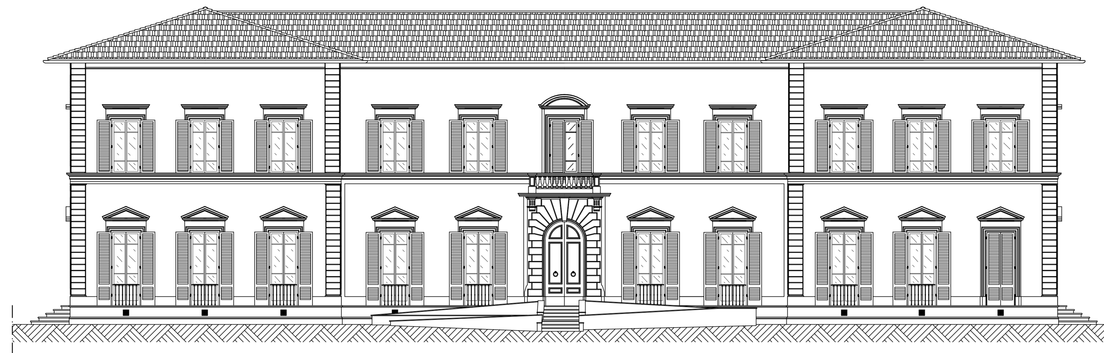
PROSPETTO FRONTALE
