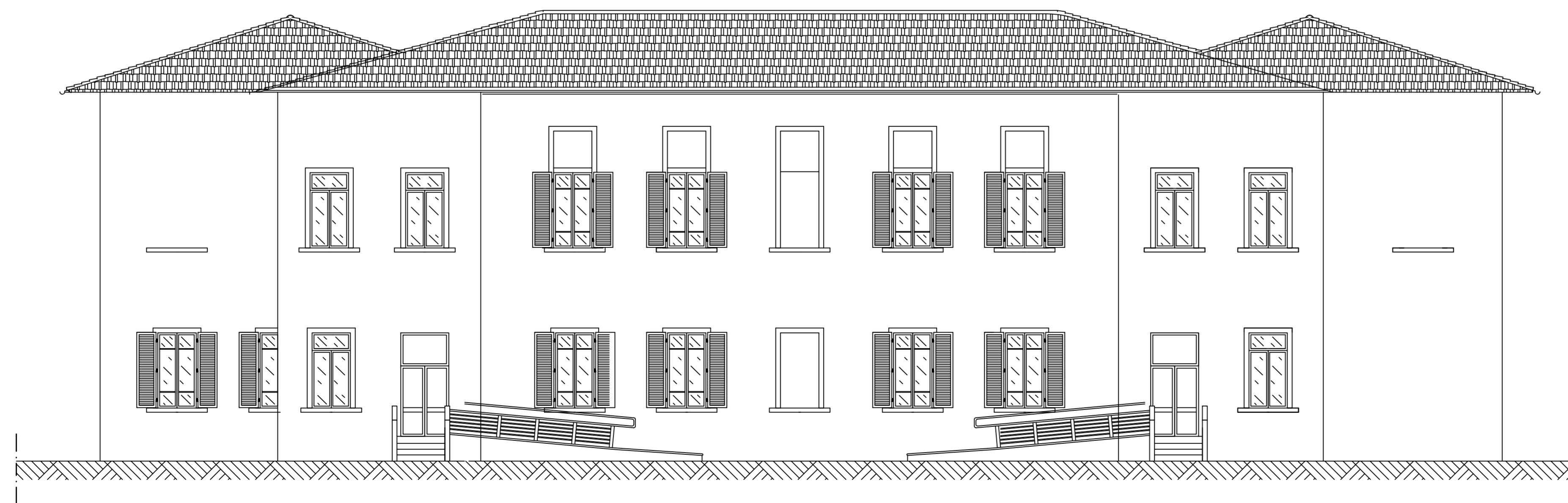
PROSPETTO TERGALE
