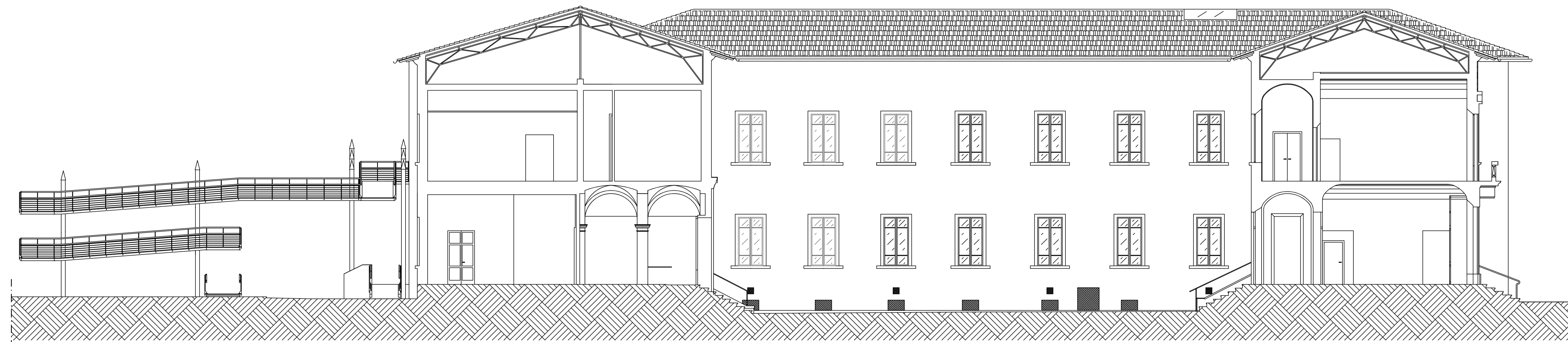
sezione D - D'
