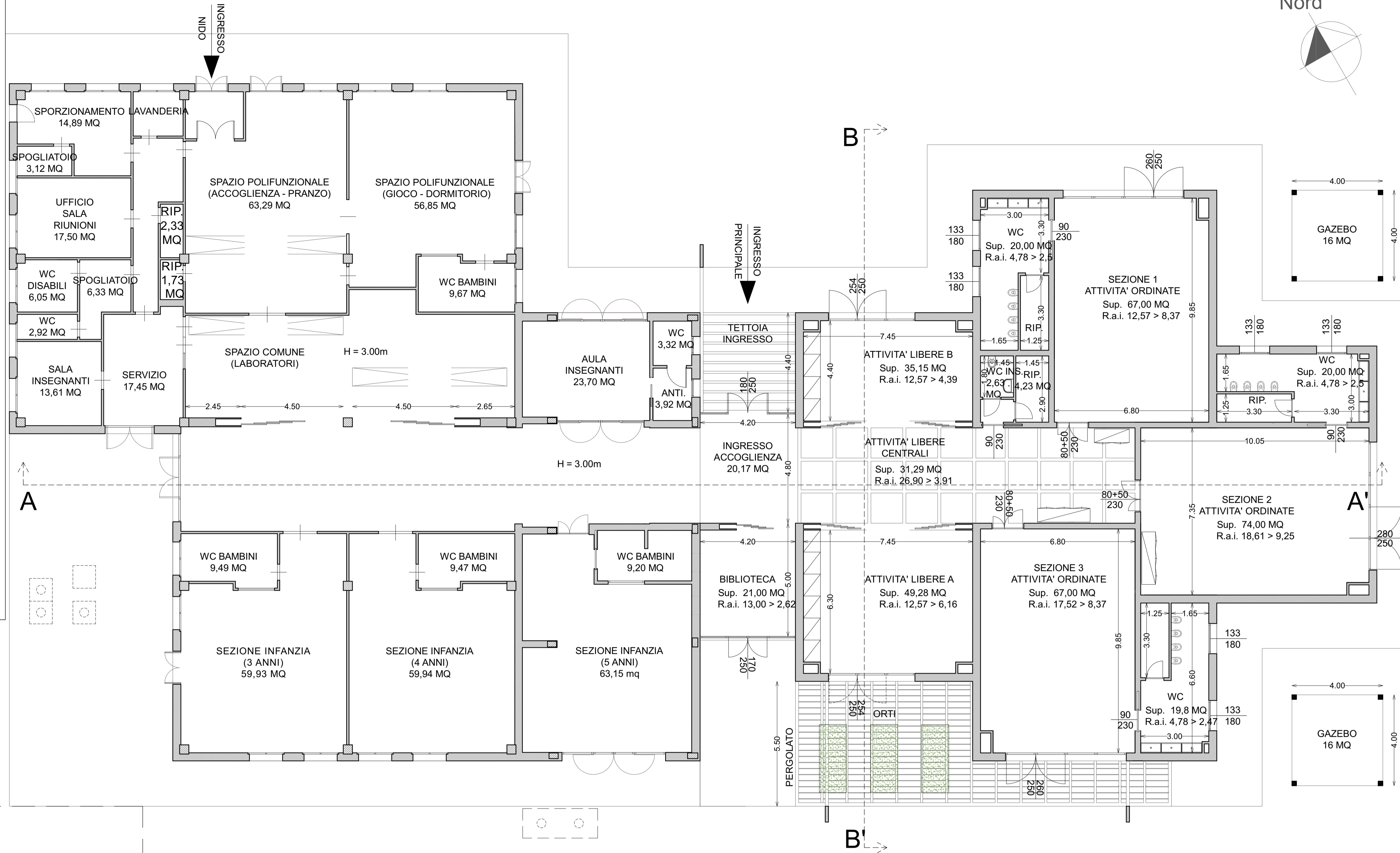
Pianta Stato di progetto, scala 1/100
