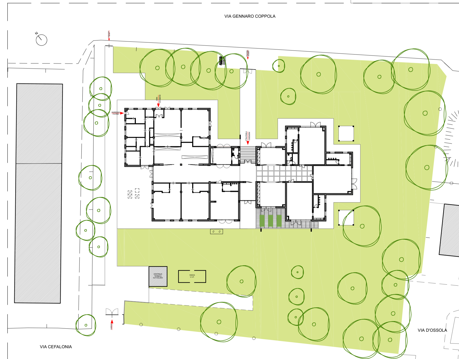
Planimetria generale Stato di progetto, scala 1/500
