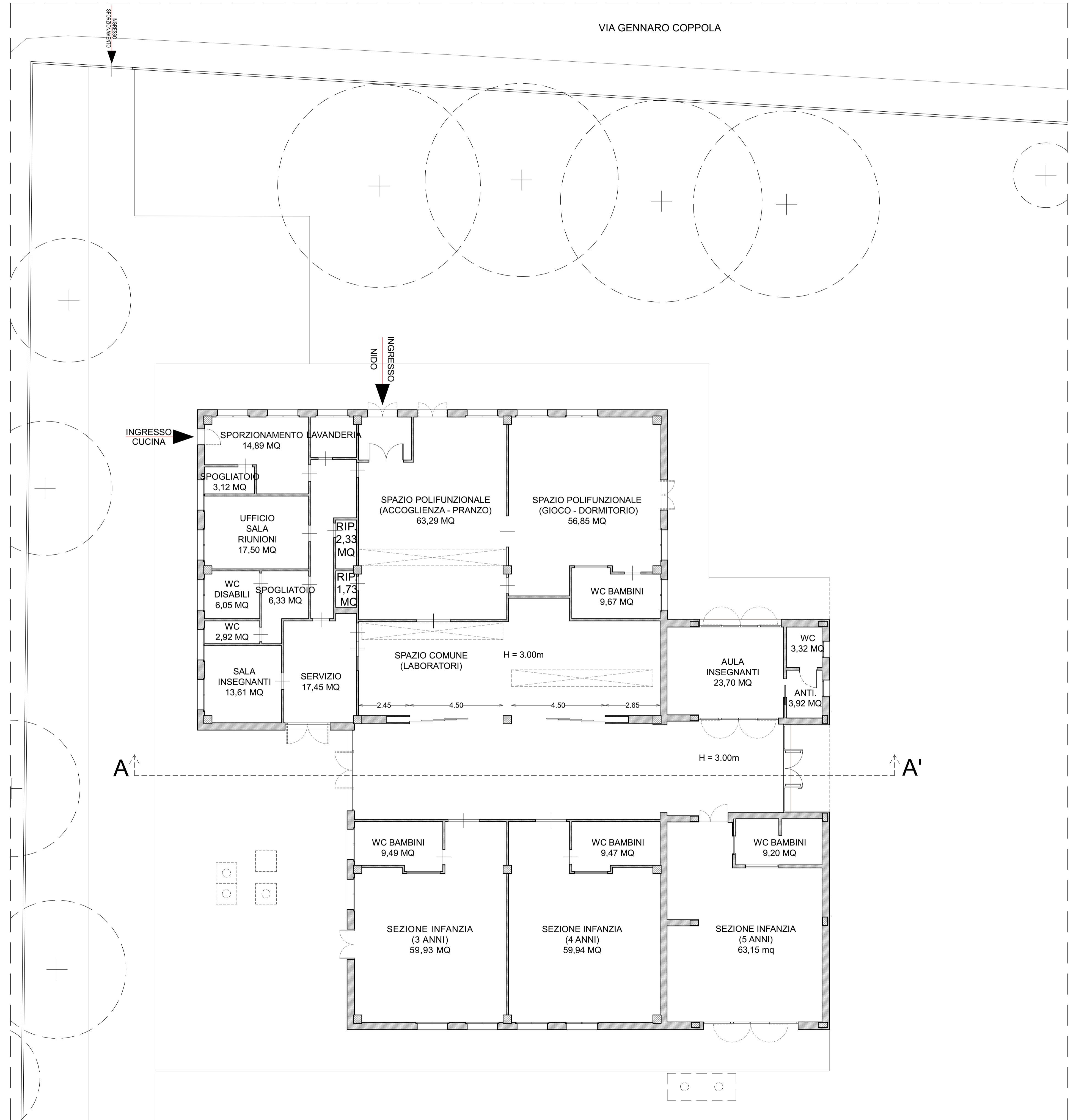
Pianta Stato attuale, scala 1/100
