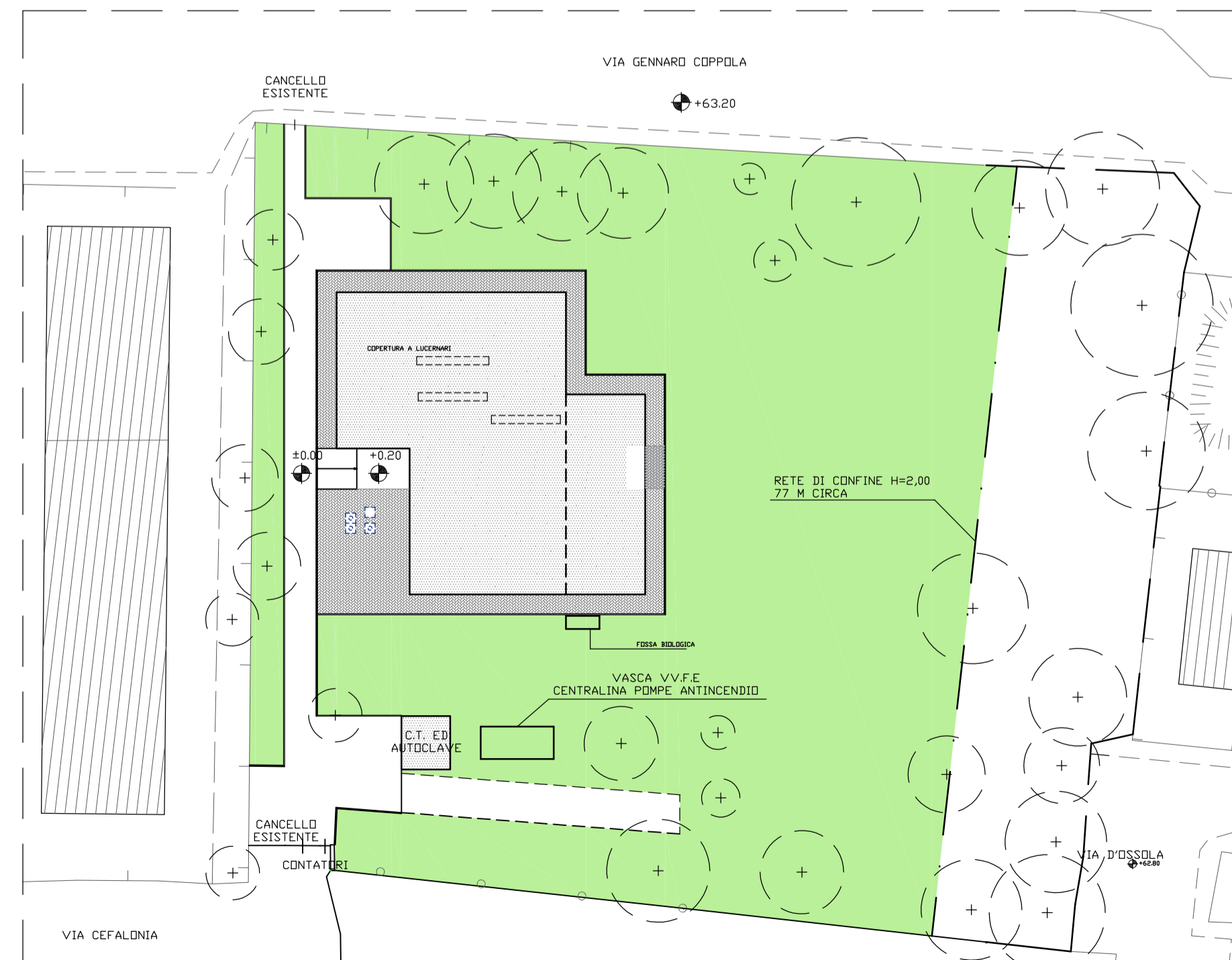
Planimetria generale Stato attuale, scala 1/500
