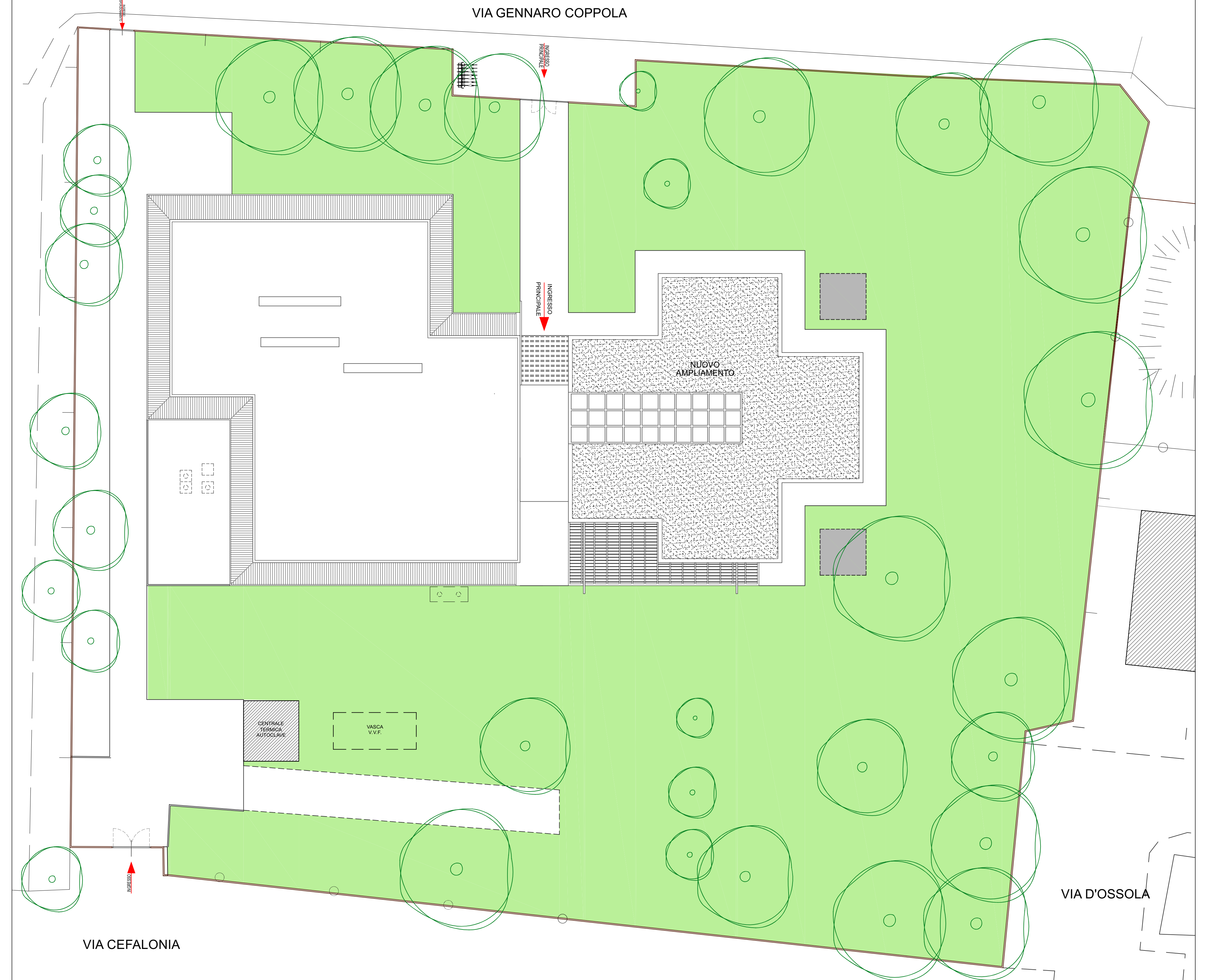
Planimetria generale di progetto, scala 1/500
