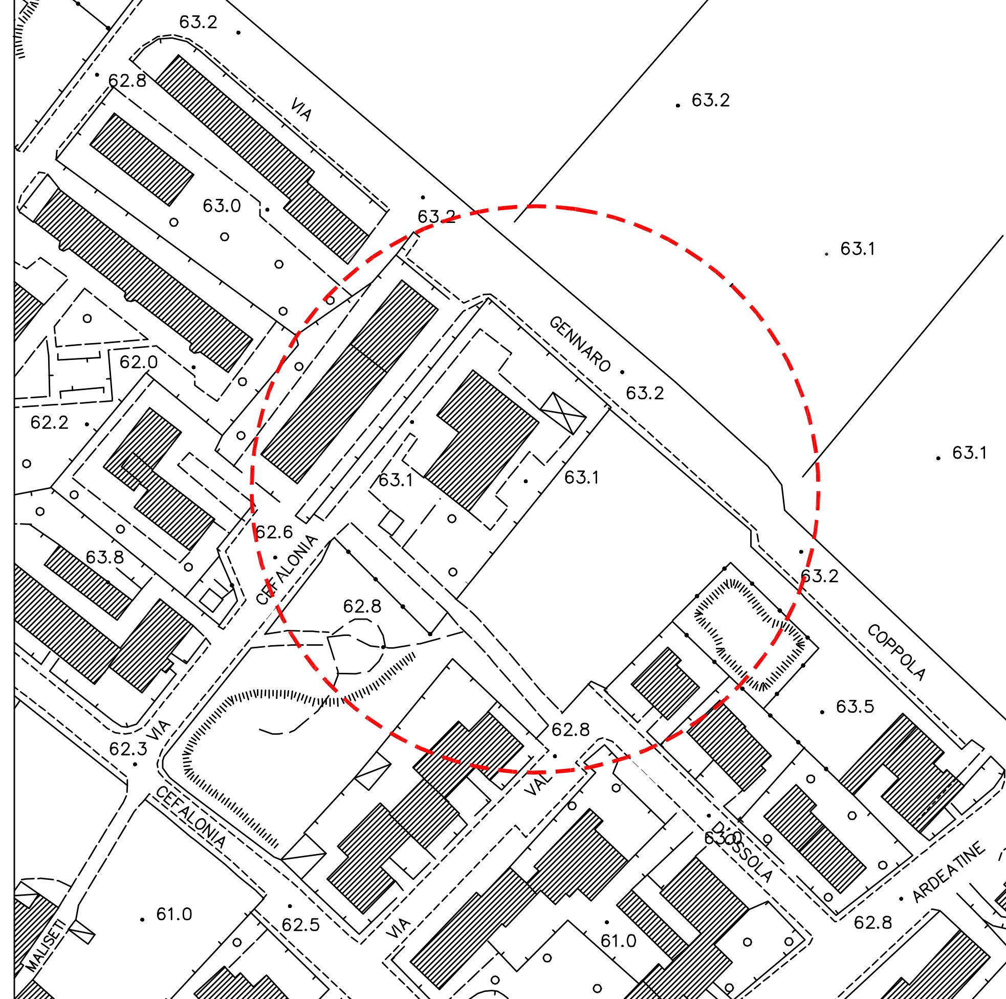
Planimetria irtef, scala 1/1000 Via Cefalonia n.12
