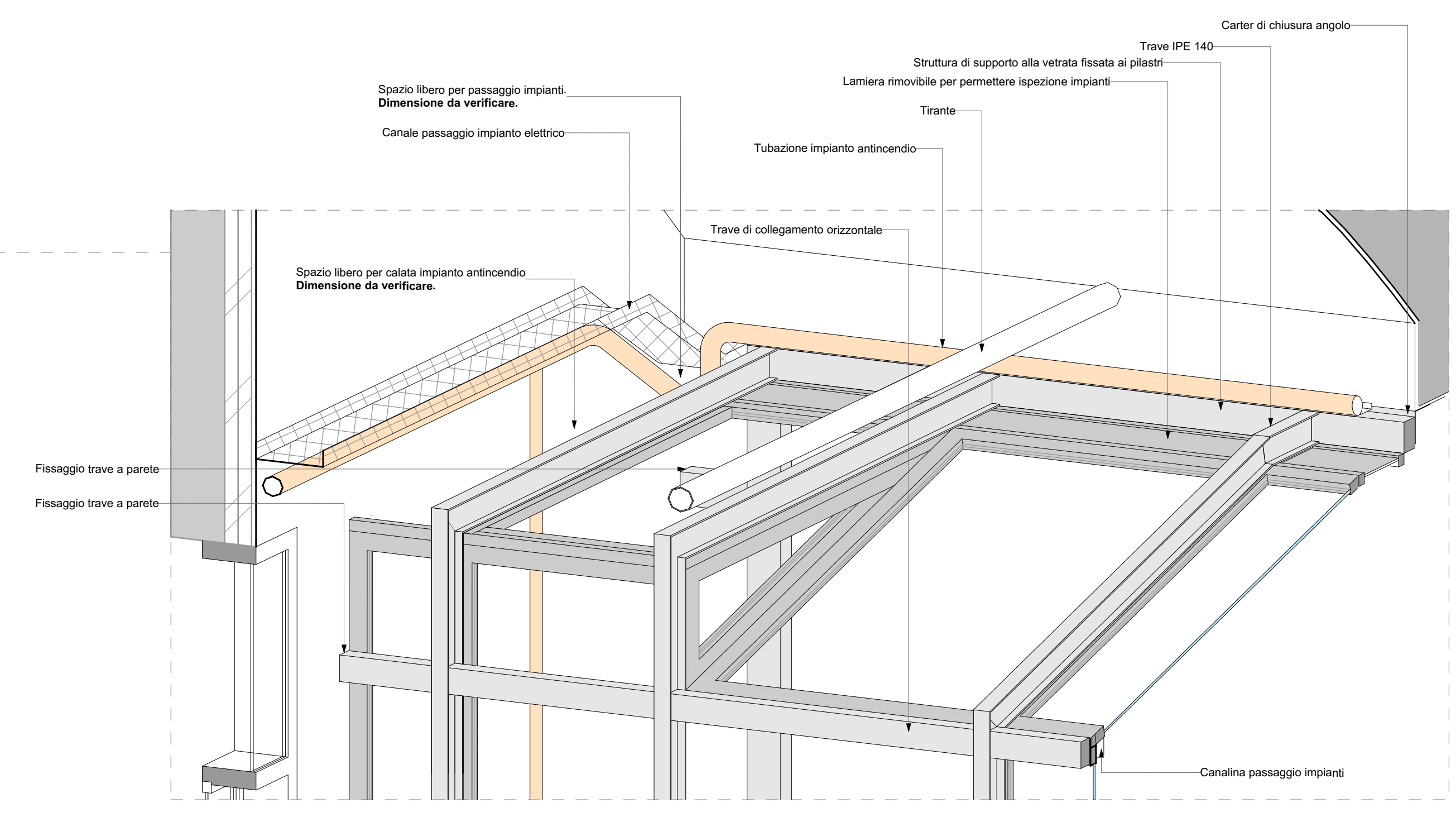
ASSONOMETRIA DI DETTAGLIO ANGOLO VETRATA
