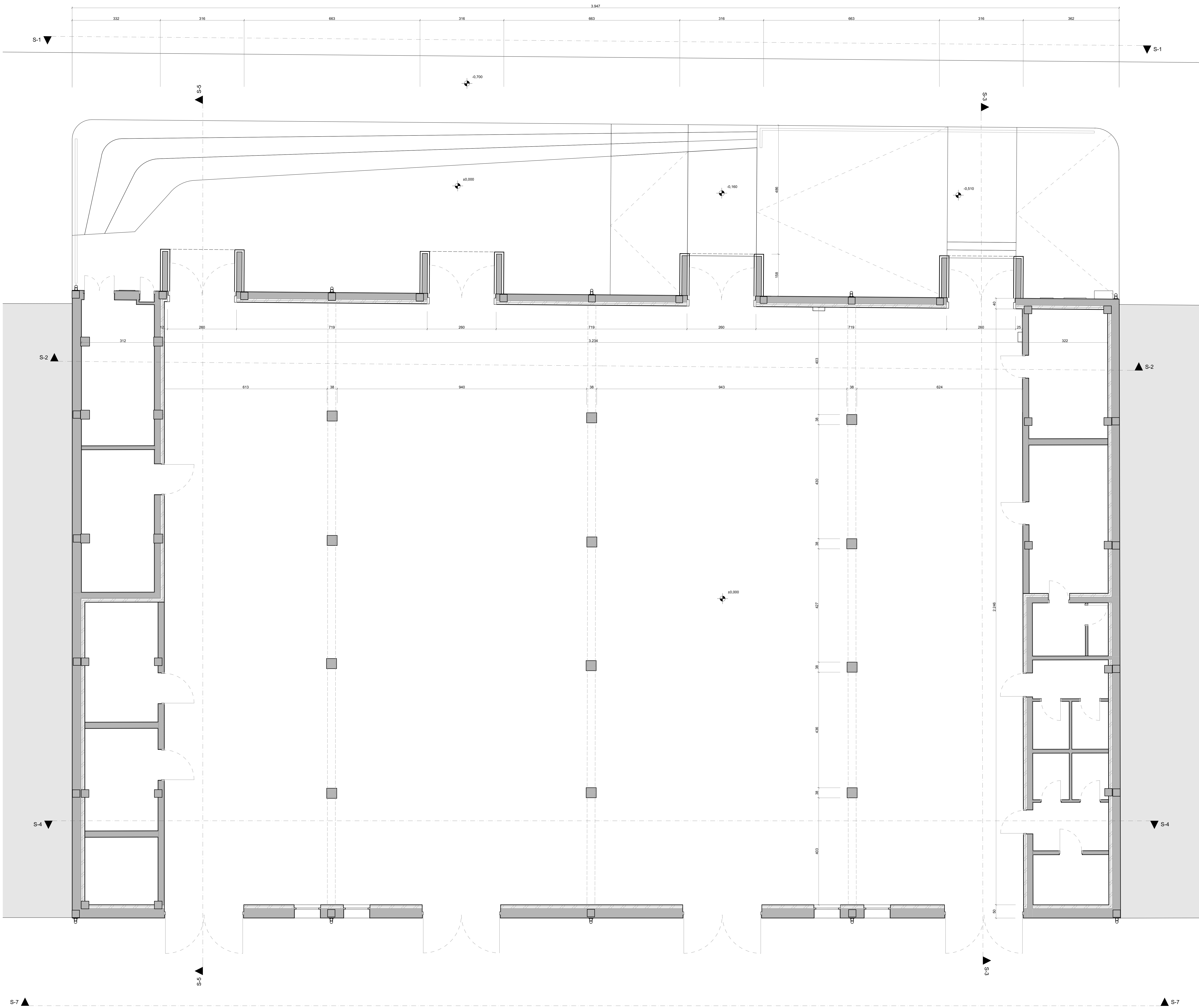
PIANTA
