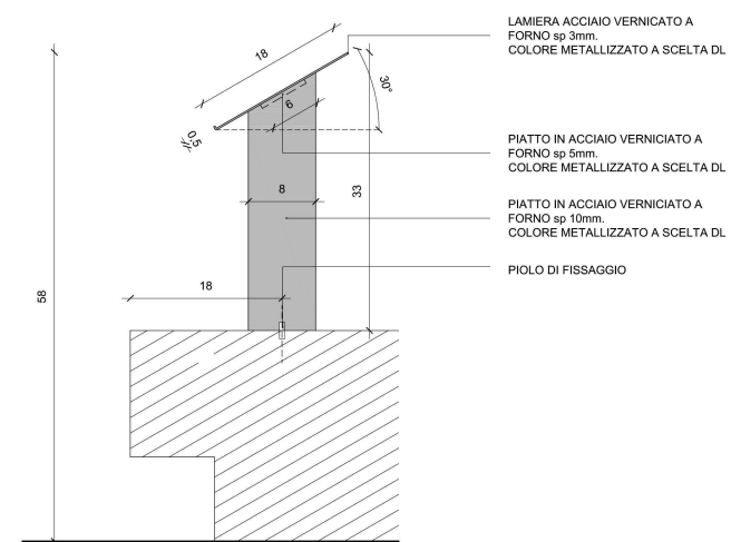
PORTADIDA PER PEDANA 1:5
