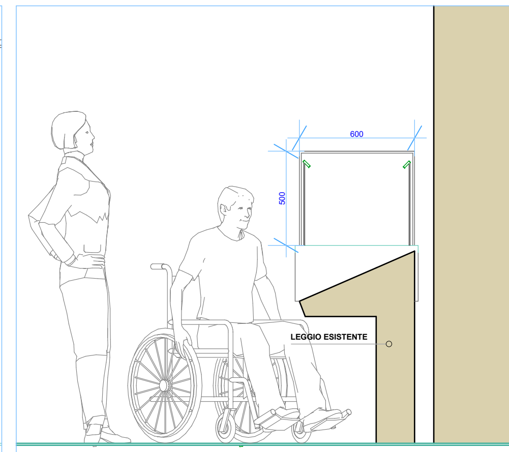
TECA IN VETRO DA REALIZZARSI IN APPOGGIO AL LEGGIO MULTIMEDIALE ESISTENTE AL PIANO TERRA, BASE IN MDF LACCATO GRIGIO, RAL MUSEO. LA CAMPANA SARA' IN VETRO 8/9 EXTRA CHIARO, FONDO RIVESTITO IN TESSUTO DI ALCANTARA CHIARO.
