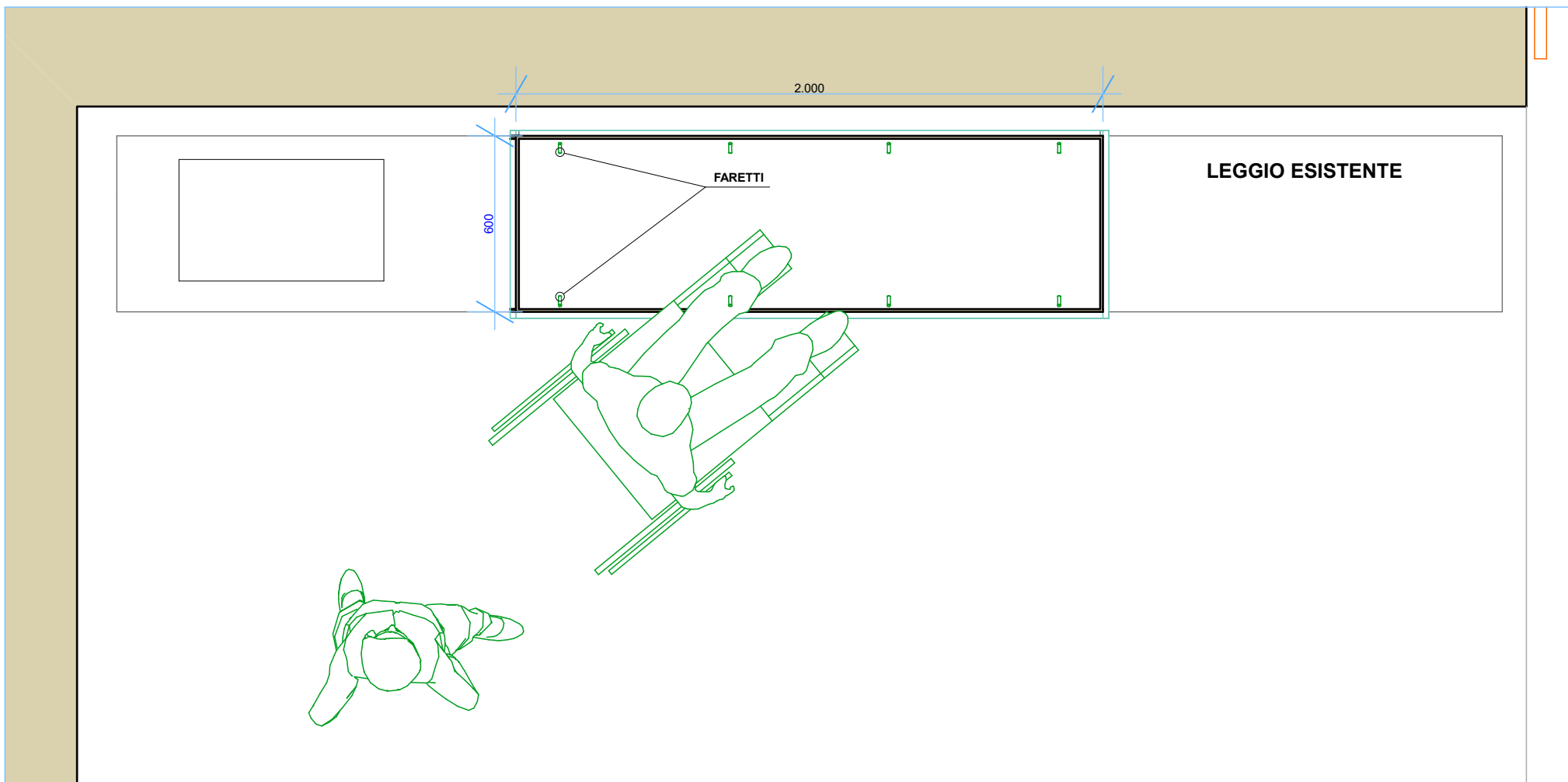
TECA IN VETRO DA REALIZZARSI IN APPOGGIO AL LEGGIO MULTIMEDIALE ESISTENTE AL PIANO TERRA, BASE IN MDF LACCATO GRIGIO, RAL MUSEO. LA CAMPANA SARA' IN VETRO 8/9 EXTRA CHIARO, FONDO RIVESTITO IN TESSUTO DI ALCANTARA CHIARO.
