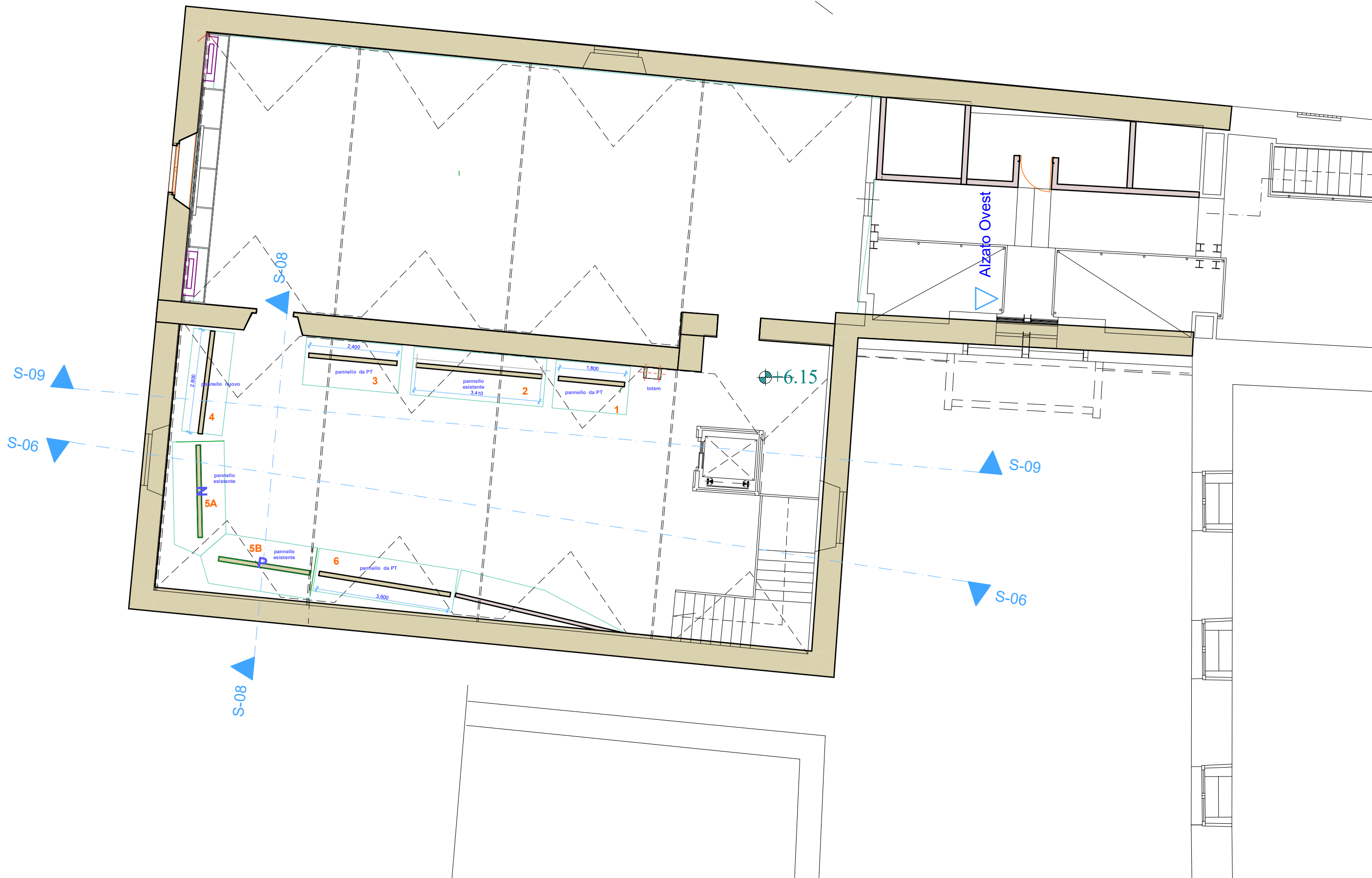
TAV.06 PLANIMETRIA ALLESTIMENTO 1° PIANO SCALA 1:100
