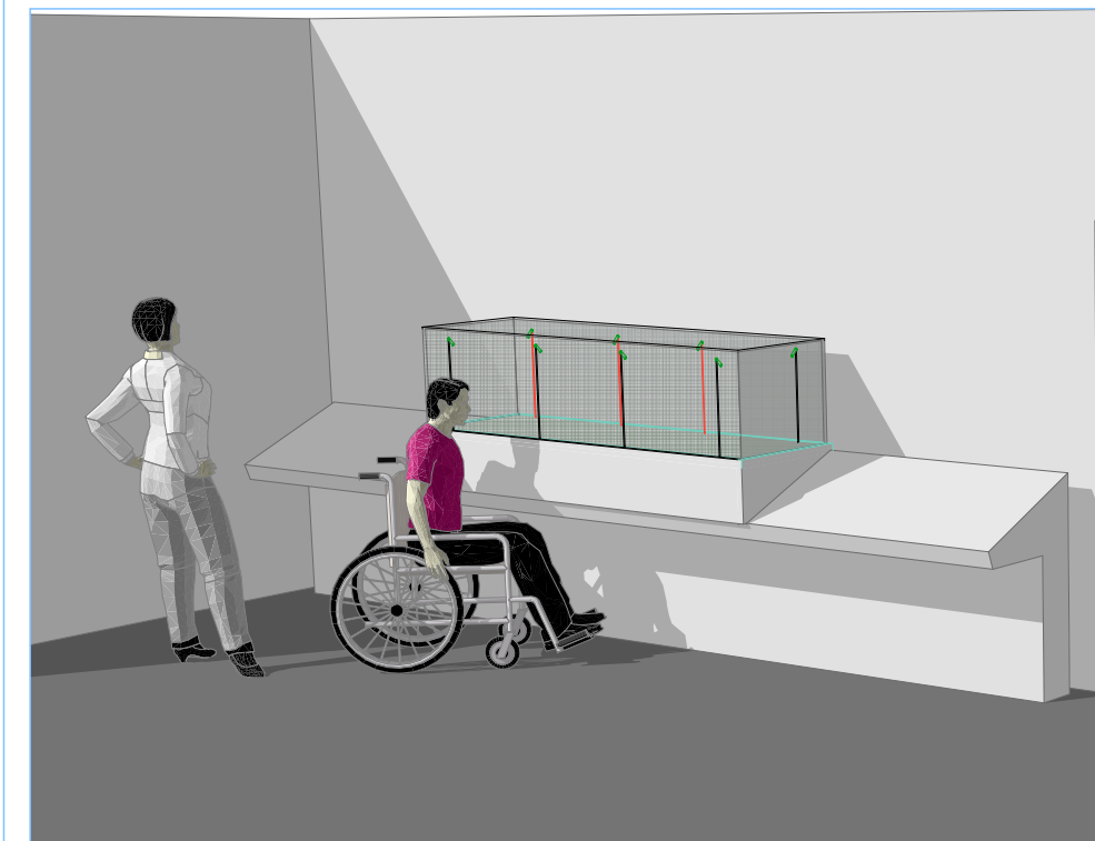
TECA IN VETRO DA REALIZZARSI IN APPOGGIO AL LEGGIO MULTIMEDIALE ESISTENTE AL PIANO TERRA, BASE IN MDF LACCATO GRIGIO, RAL MUSEO. LA CAMPANA SARA' IN VETRO 8/9 EXTRA CHIARO, FONDO RIVESTITO IN TESSUTO DI ALCANTARA CHIARO.
