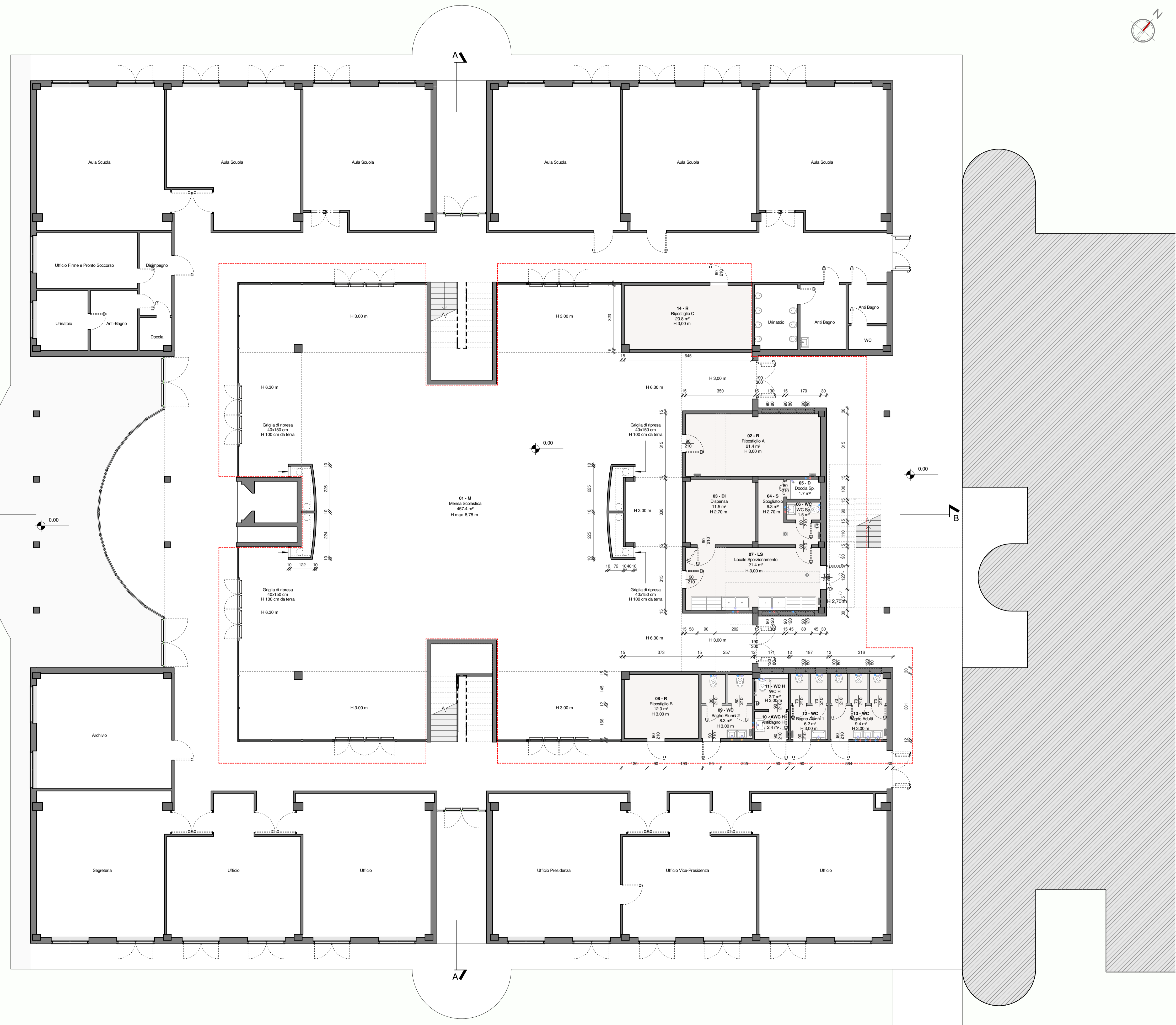
STATO DI PROGETTO - Pianta Piano Terra - SCALA 1:100
