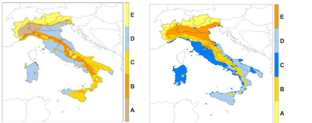
Figura 8: Mappa delle anomalie, scenario RCP8.5, confronto simulazioni 2021 - 2050 e 1981 - 2010
