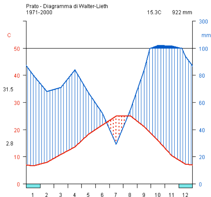
Figura 5: Diagrammi di Walter-Lieth
