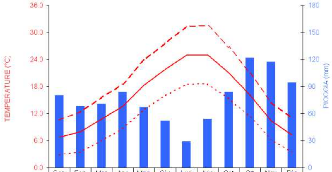
Diagramma Termo-Pluviometrico PRATO (medie 1971-2000)
