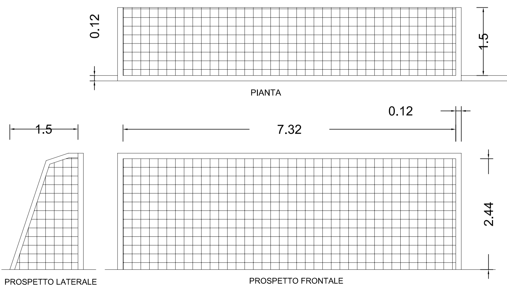
DETTAGLIO PORTA DA CALCIO - SCALA 1:50
