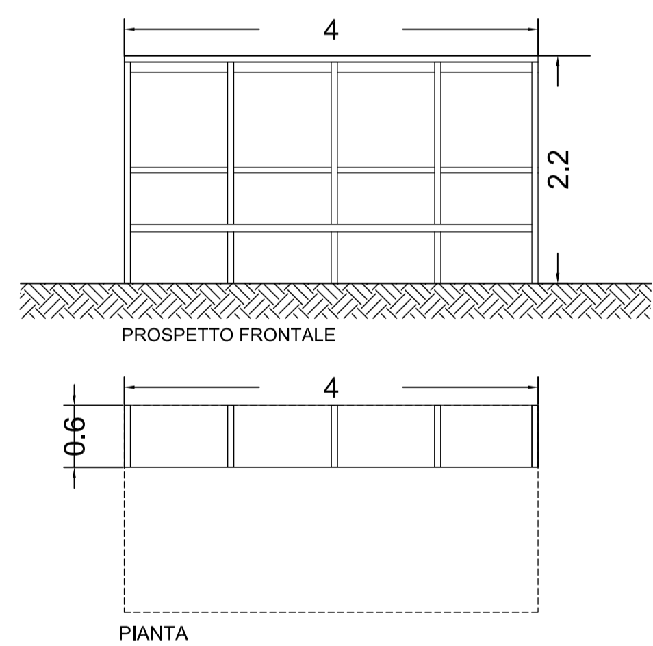
DETTAGLIO F - SCALA 1:50
