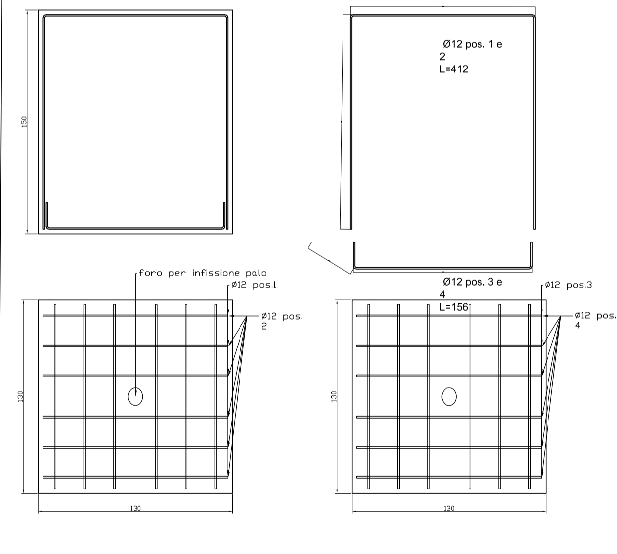
DETTAGLIO C - plinto palo porta da rugby
