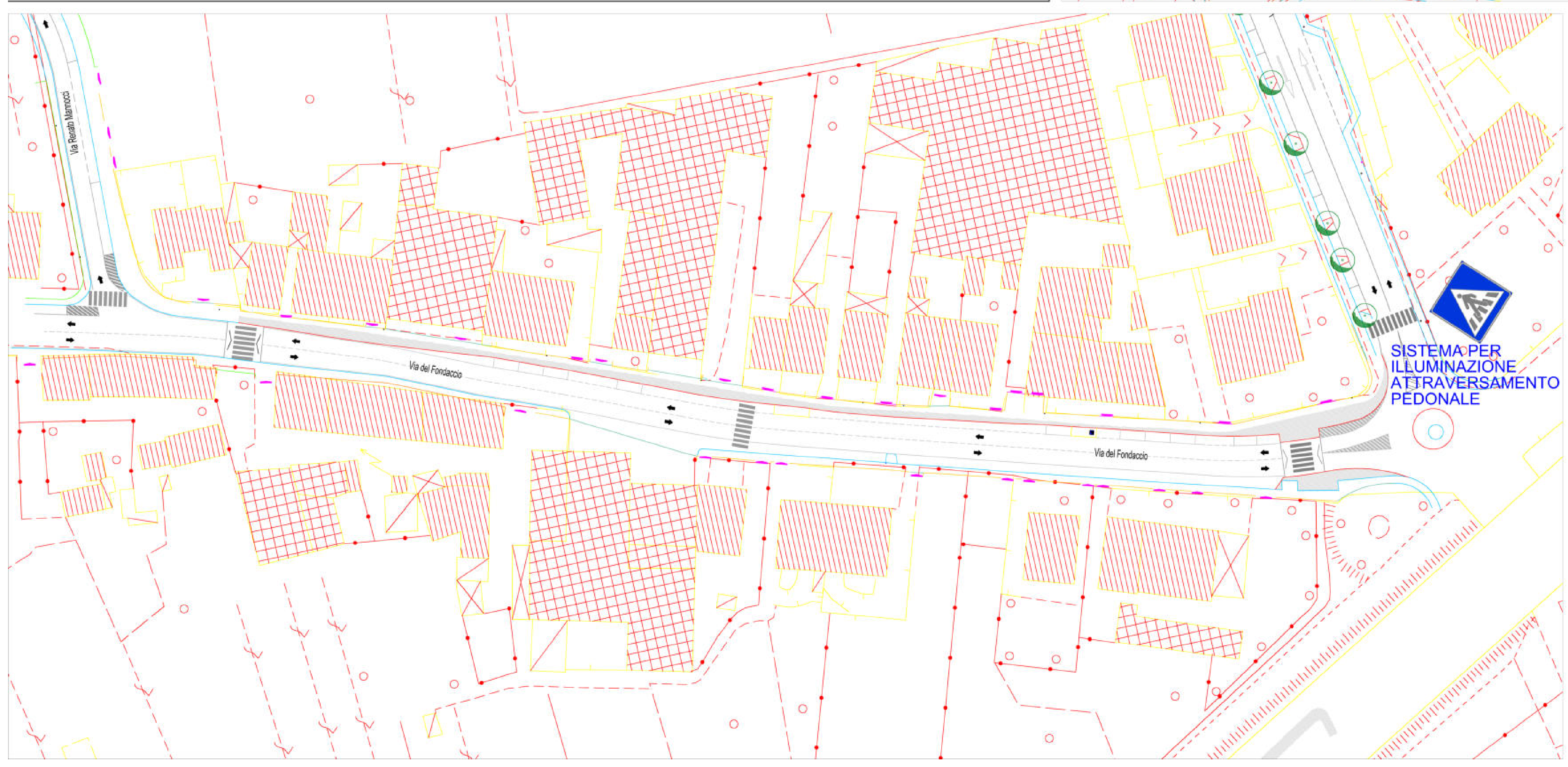
SISTEMA PER ILLUMINAZIONE ATTRAVERSAMENTO PEDONALE SCHEMA E PARTICOLARE PALI
