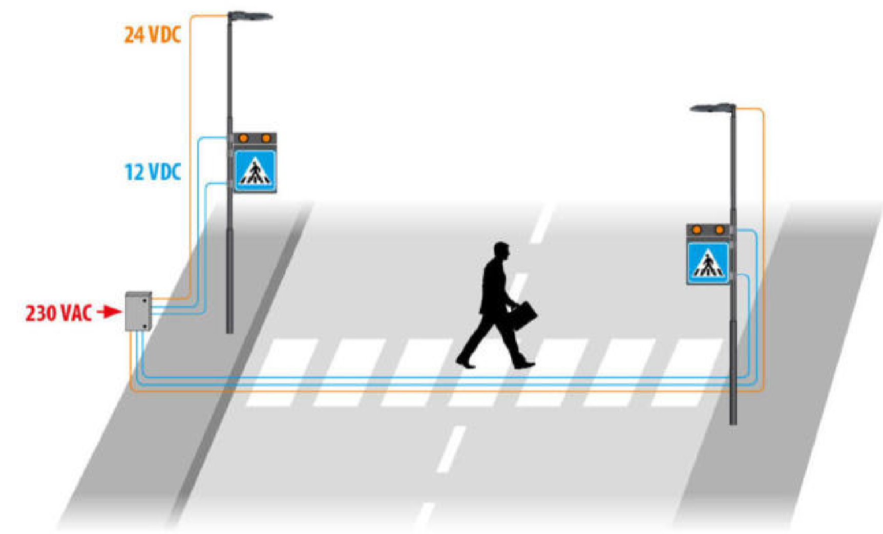
SISTEMA PER ILLUMINAZIONE ATTRAVERSAMENTO PEDONALE SCHEMA E PARTICOLARE PALI
