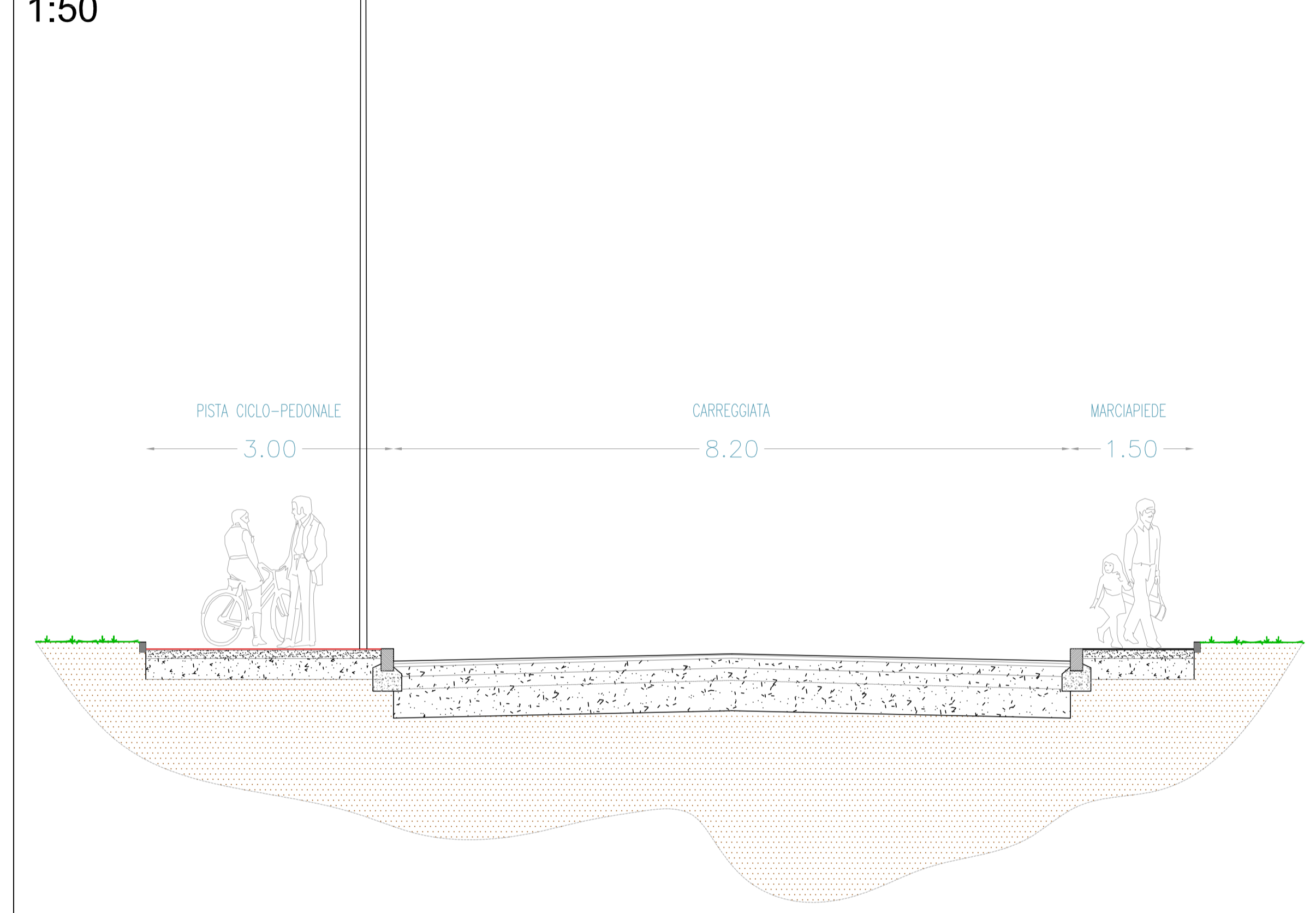
SEZIONE 3-3 - PISTA CICLOPEDONALE - VIA S. MARTINO PER GALCETI 1:50
