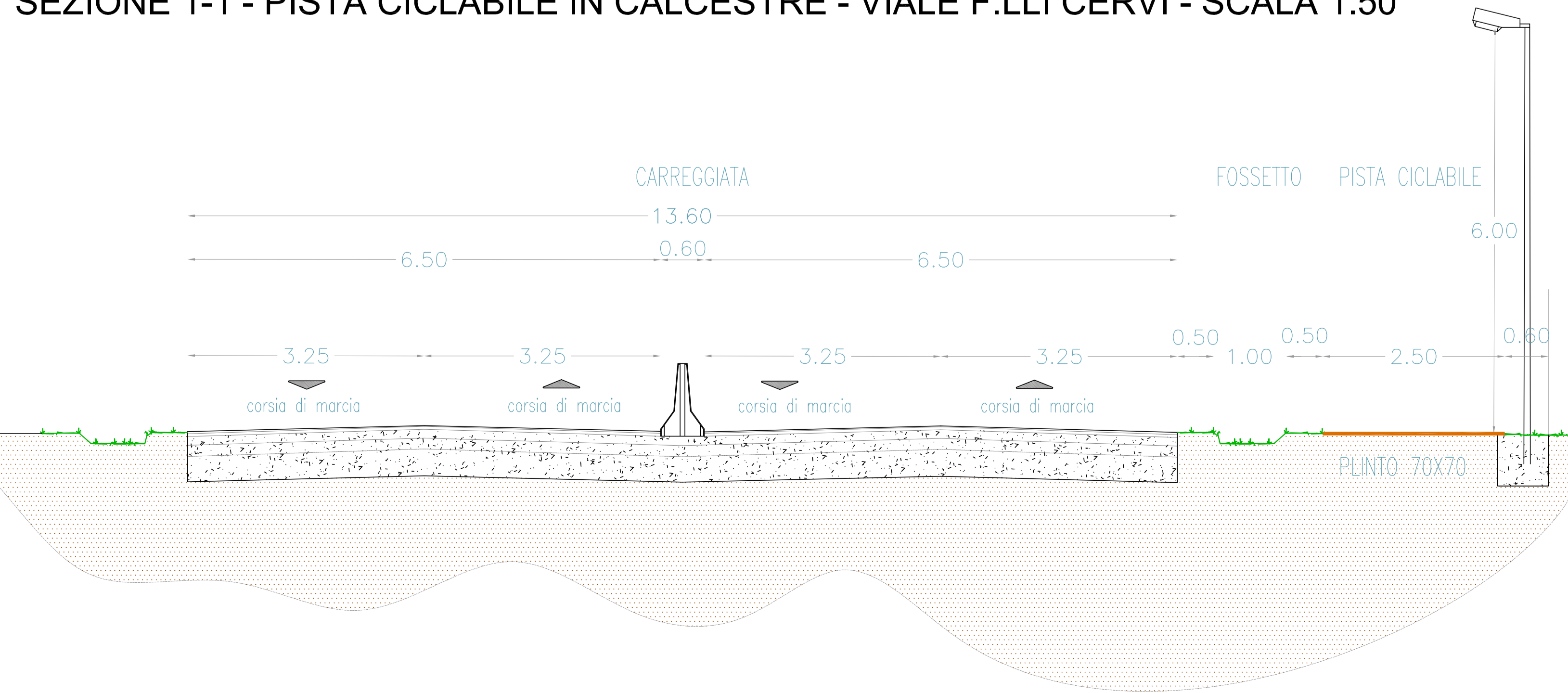
SEZIONE 1-1 - PISTA CICLABILE IN CALCESTRE - VIALE F.LLI CERVI - SCALA 1:50
