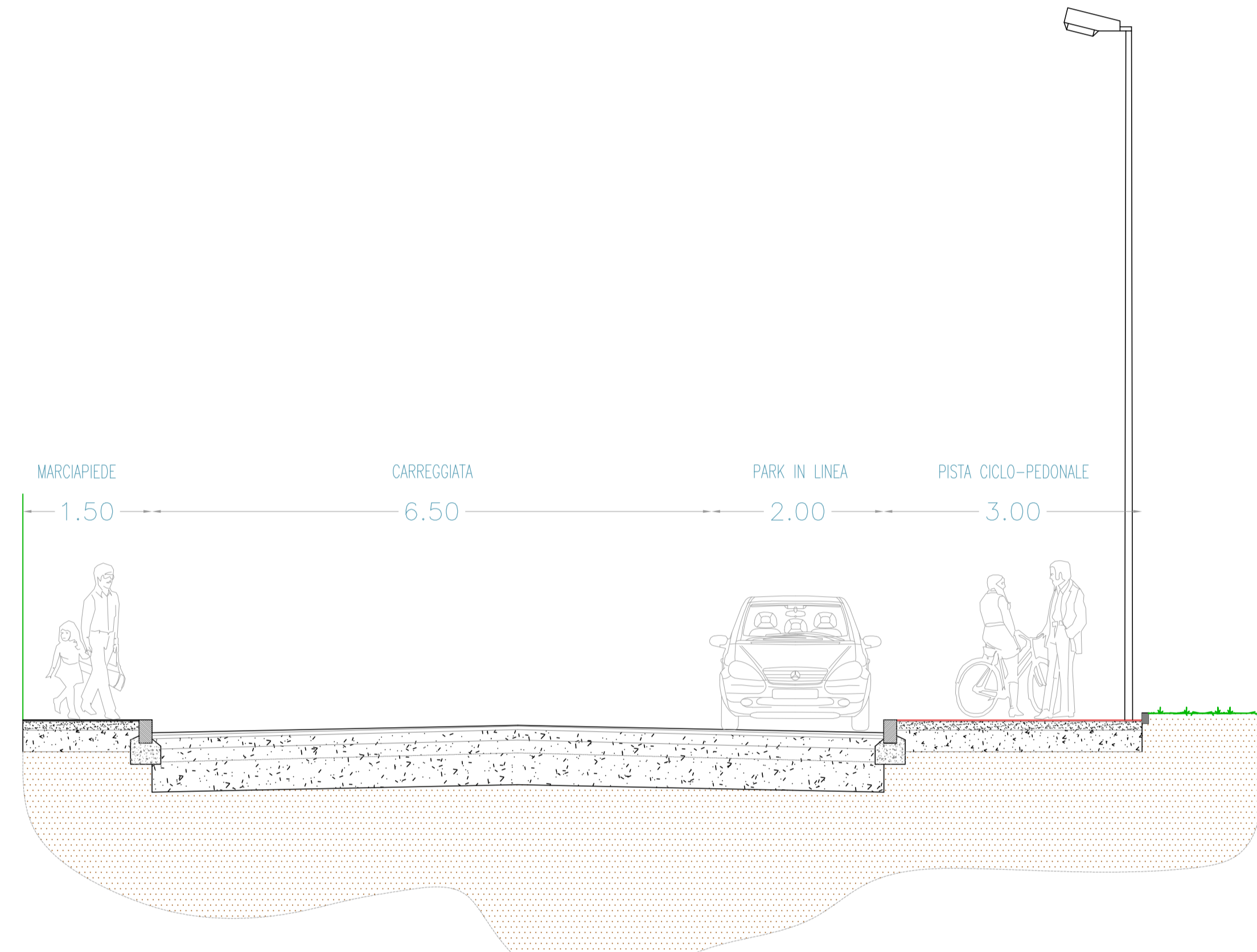
SEZIONE 2-2 - PISTA CICLOPEDONALE - VIA S. MARTINO PER GALCETI 1:50
