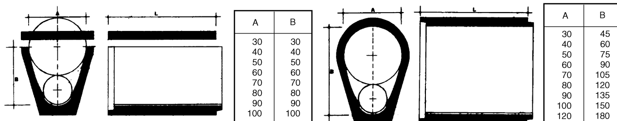
FIG. 22 - Condotti semiovoidali e ovoidali prefabbricati. Dimensioni indicative
