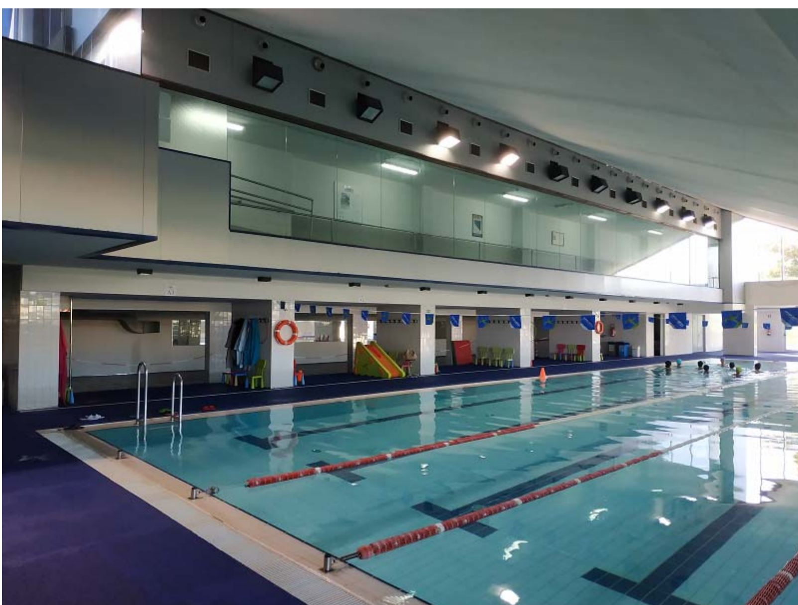
Vista ballatoio piscina con i profilati metallici su lato piscina
