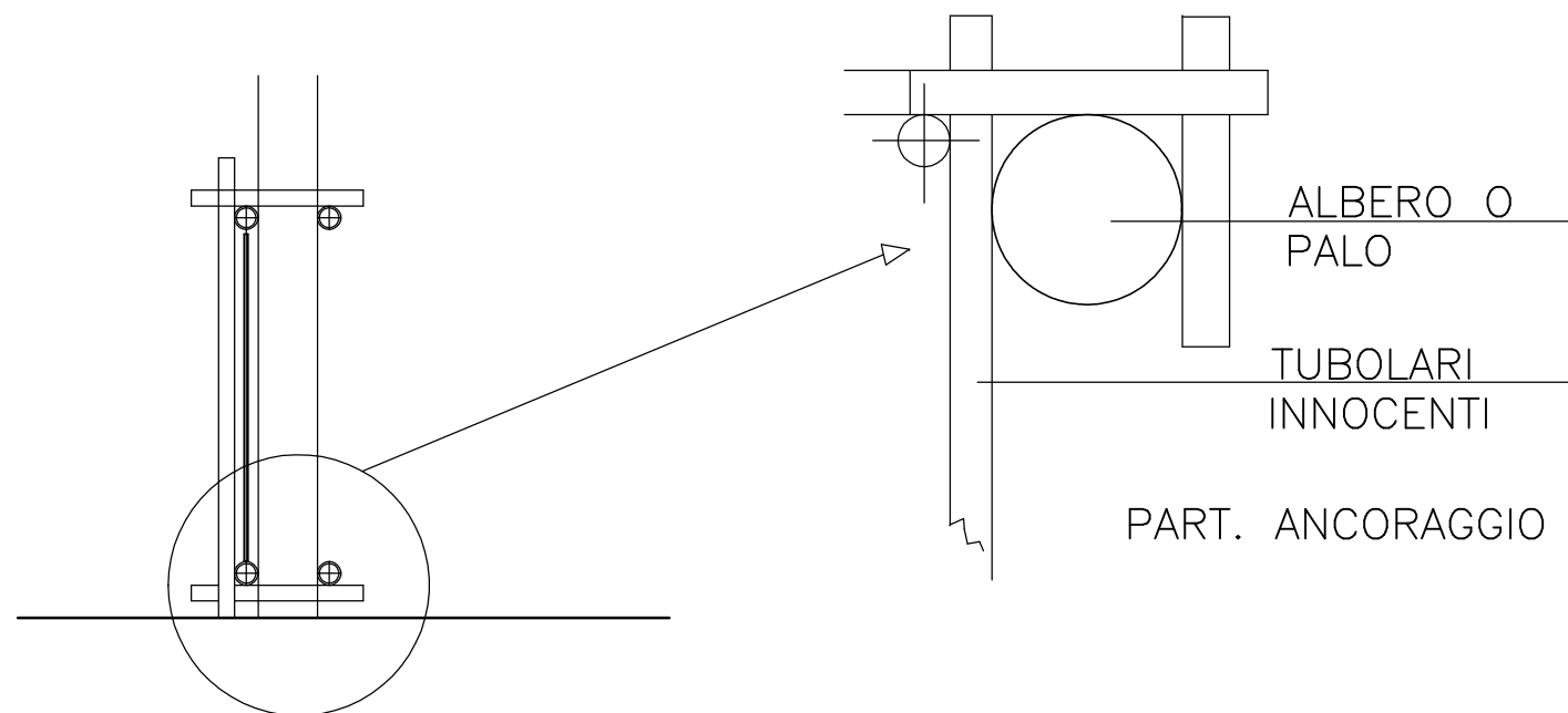
ANCORAGGIO STRUTTURA A PALO O ALBERO
