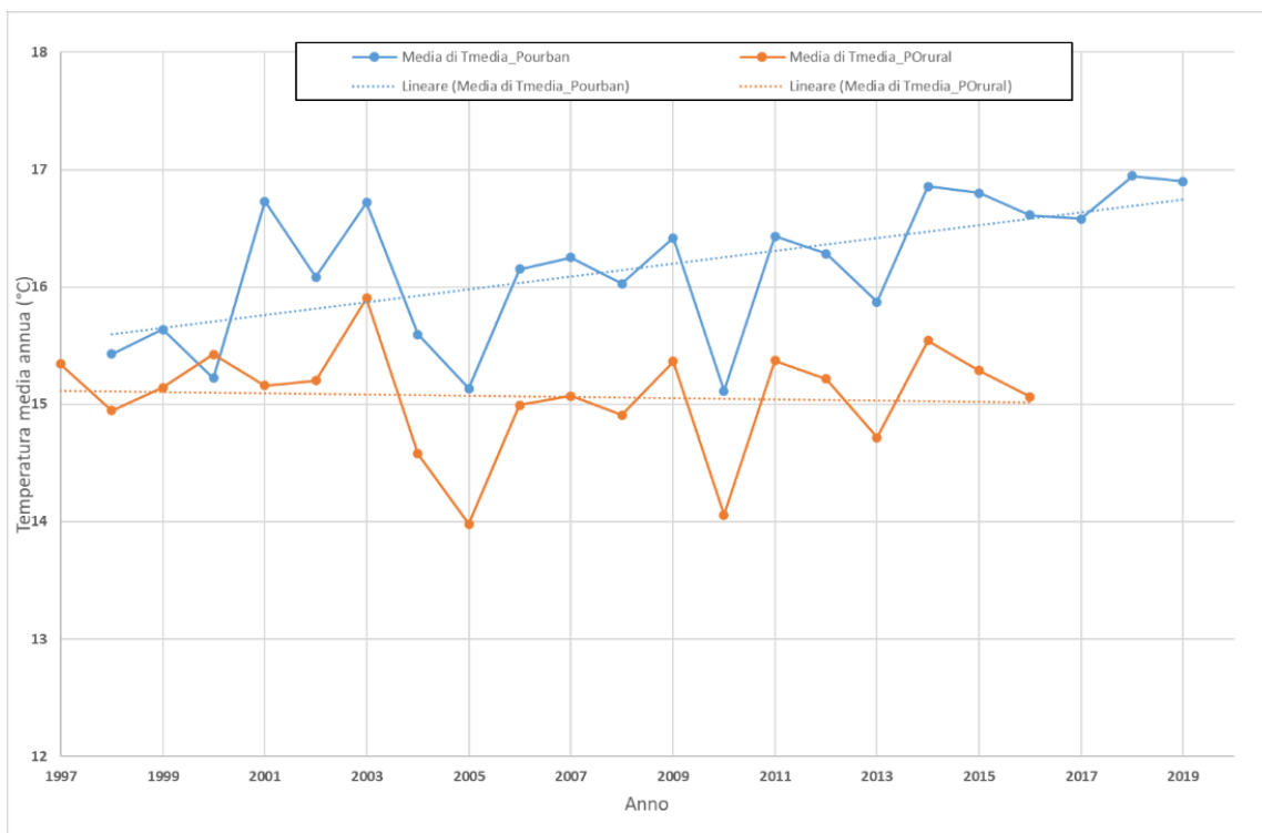
195 Figura 2. Media annuale della temperatura dell'aria per Prato_urban e Prato_rural con le loro linee di tendenza dal 196 1997 al 2019.
