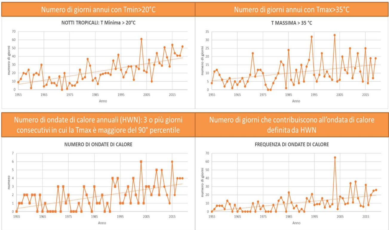
294 Figura 7. Andamento degli indici climatici notti tropicali, numero di giorni annui con temperatura massima > 35°C, 295 numero di ondate di calore annuale e frequenza delle ondate di calore dal 1955 al 2019 per la stazione Prato_Urban.
