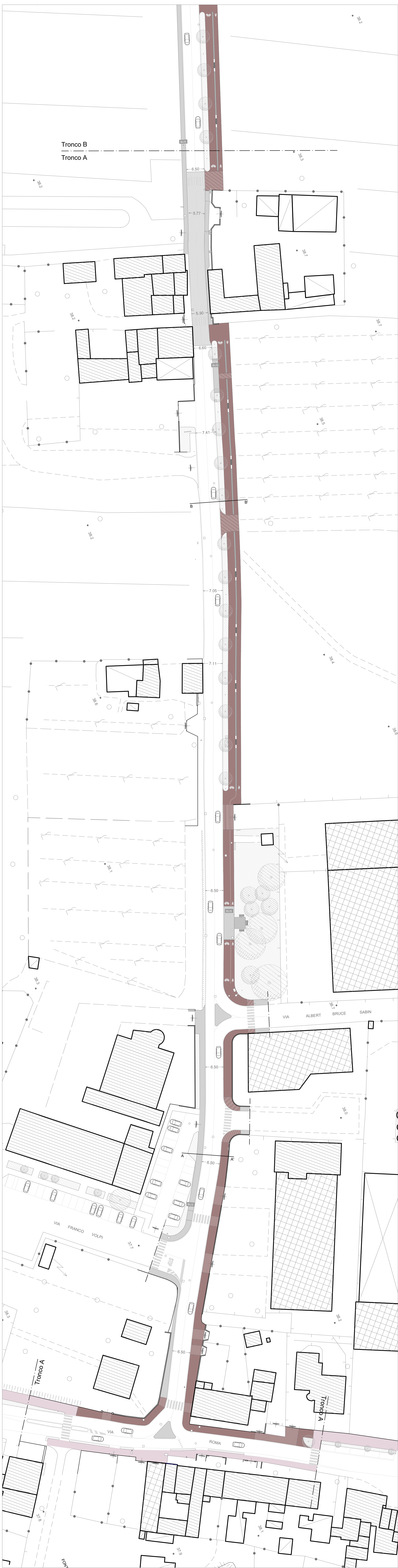
STATO DI PROGETTO, TRONCO A, scala 1:500
