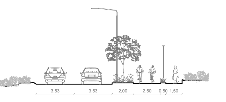
SEZIONE BB', scala 1:200
