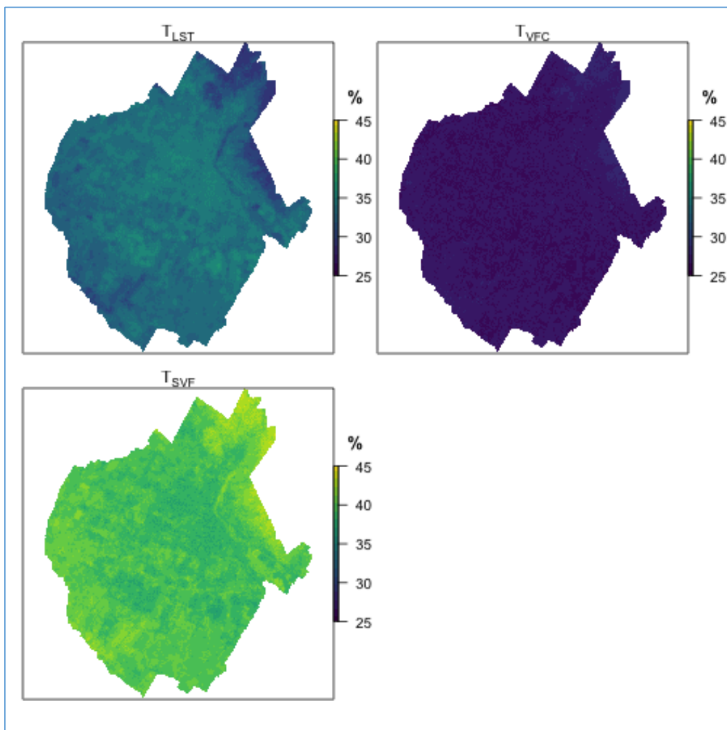
617 618 Figura 27. Contributo percentuale dei layer T_{LST} e T_{VFC} e T_{SVF} al calcolo dell'indice UHTI.
