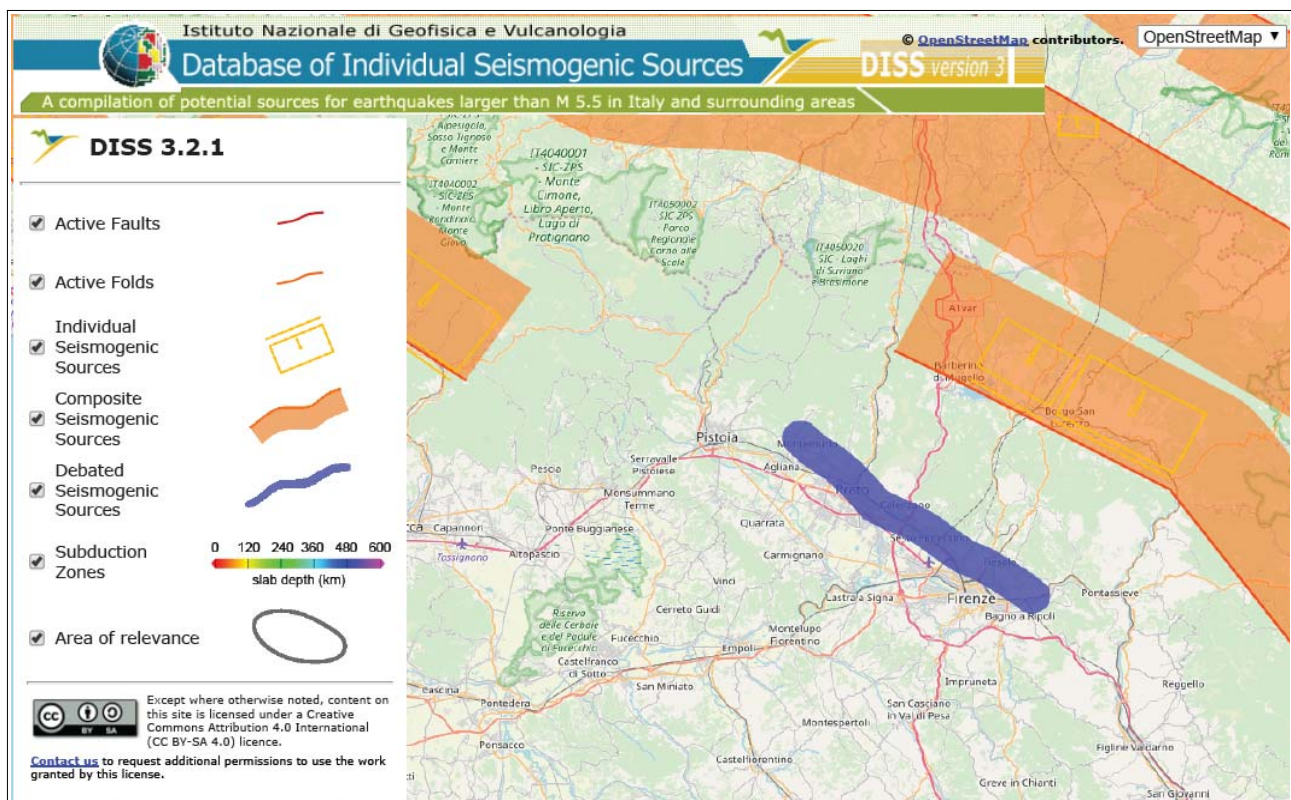
figura 6- mappa delle aree sismogenetiche di interesse (Fonte: Database of Individual Seismogenic Sources - DISS 3 - http://diss.rm.ingv.it/diss/ )
