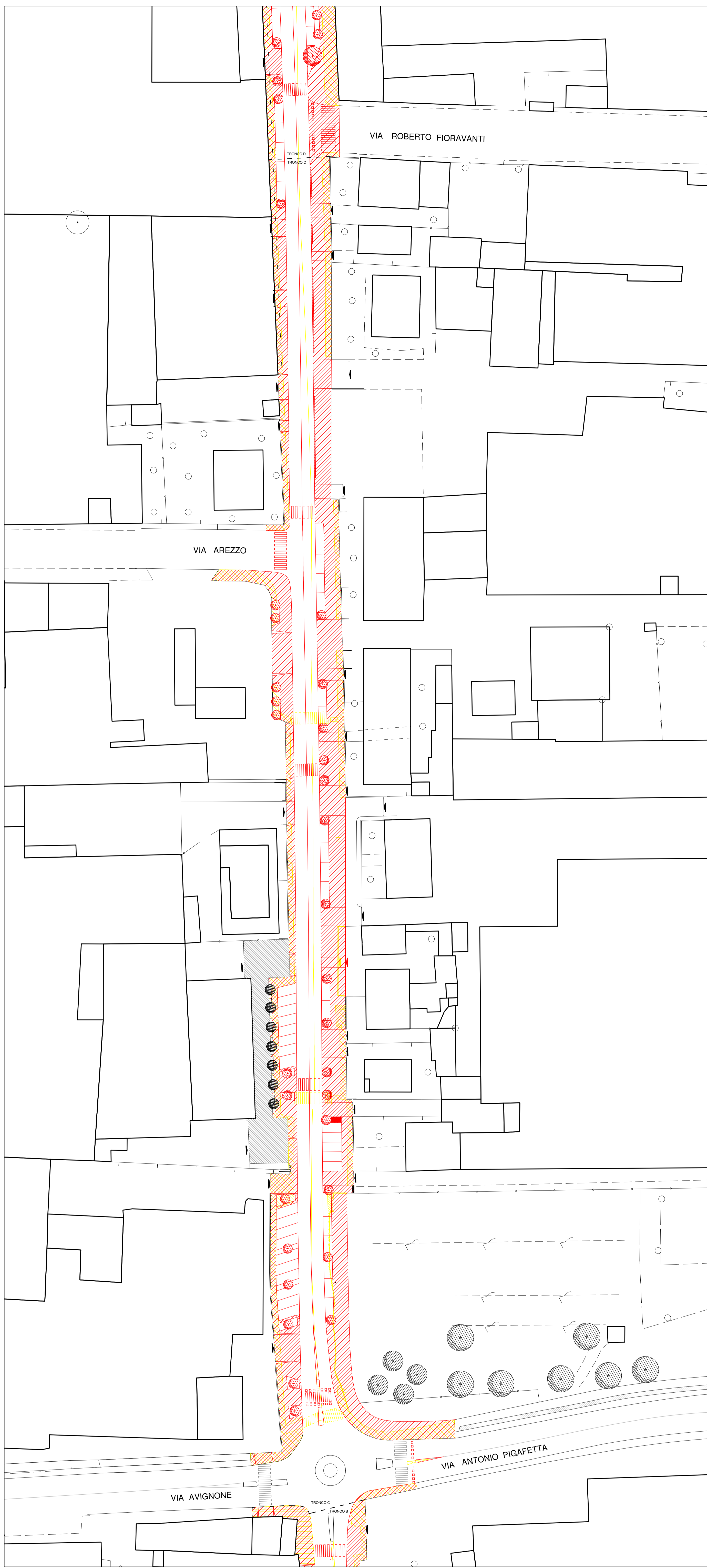
STATO SOVRAPPOSTO, TRONCO C, scala 1:500
