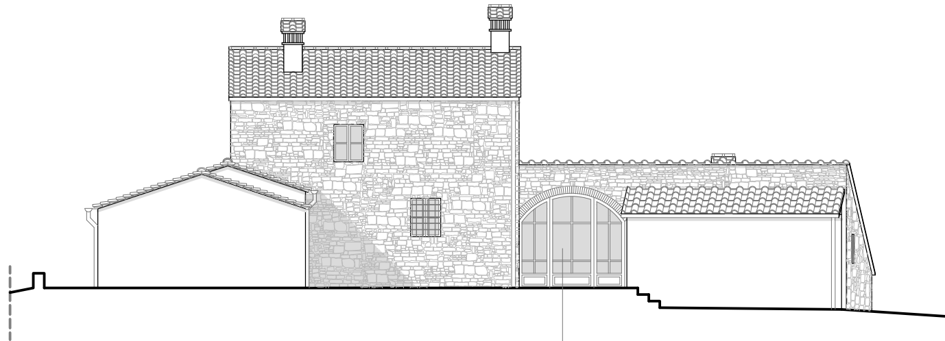
Prospetto sud-est
