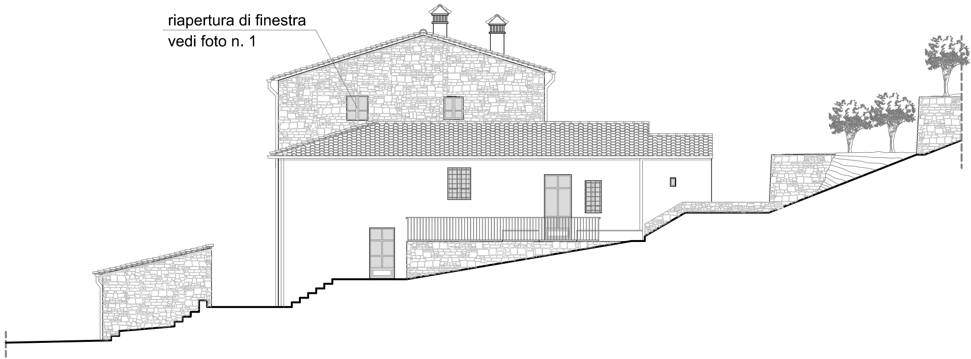
Prospetto sud-est
