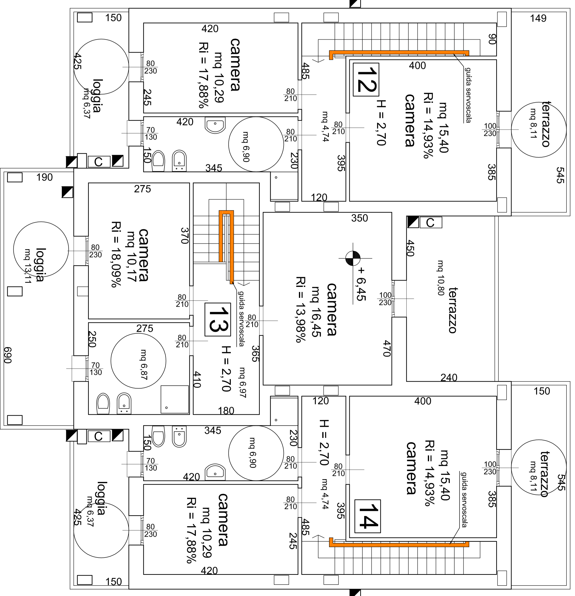
PIANTA PIANO SECONDO
