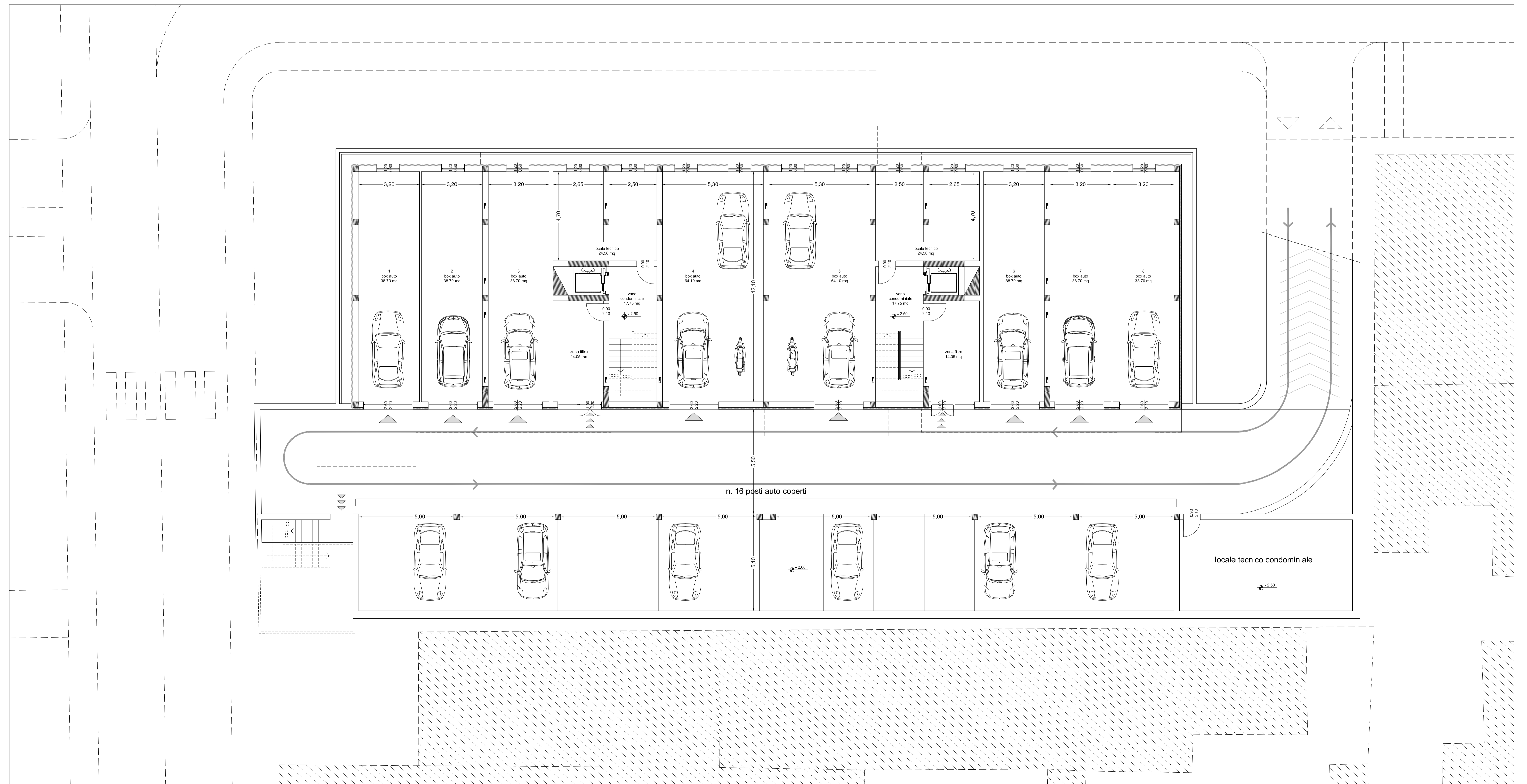
PIANTA PIANO INTERRATO
