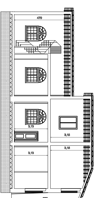
SEZIONE C-C
