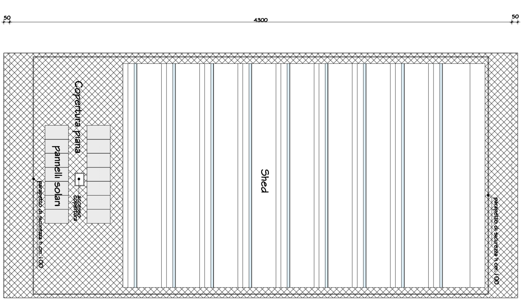
PIANTA COPERTURA
