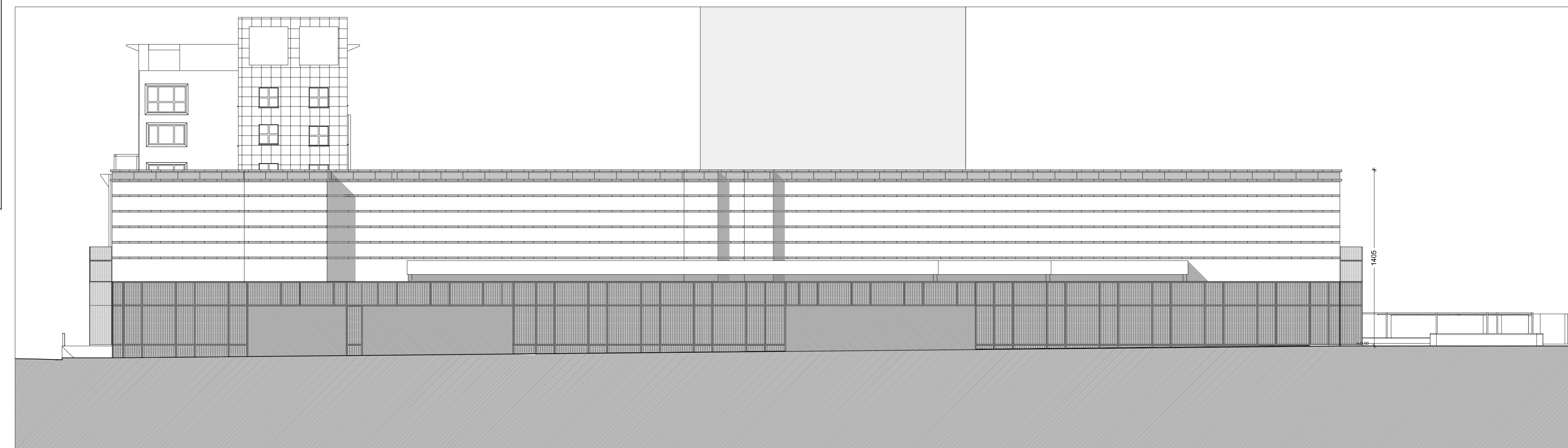
PROSPETTO EST
