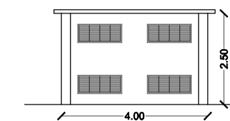
Prospetto Ovest
