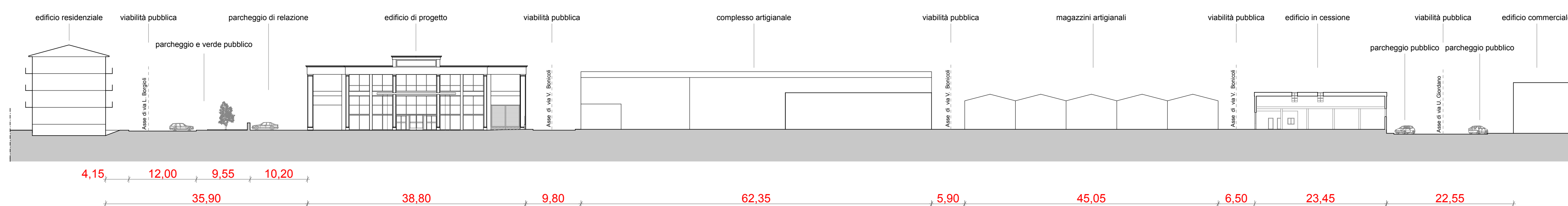
Profilo B-B
