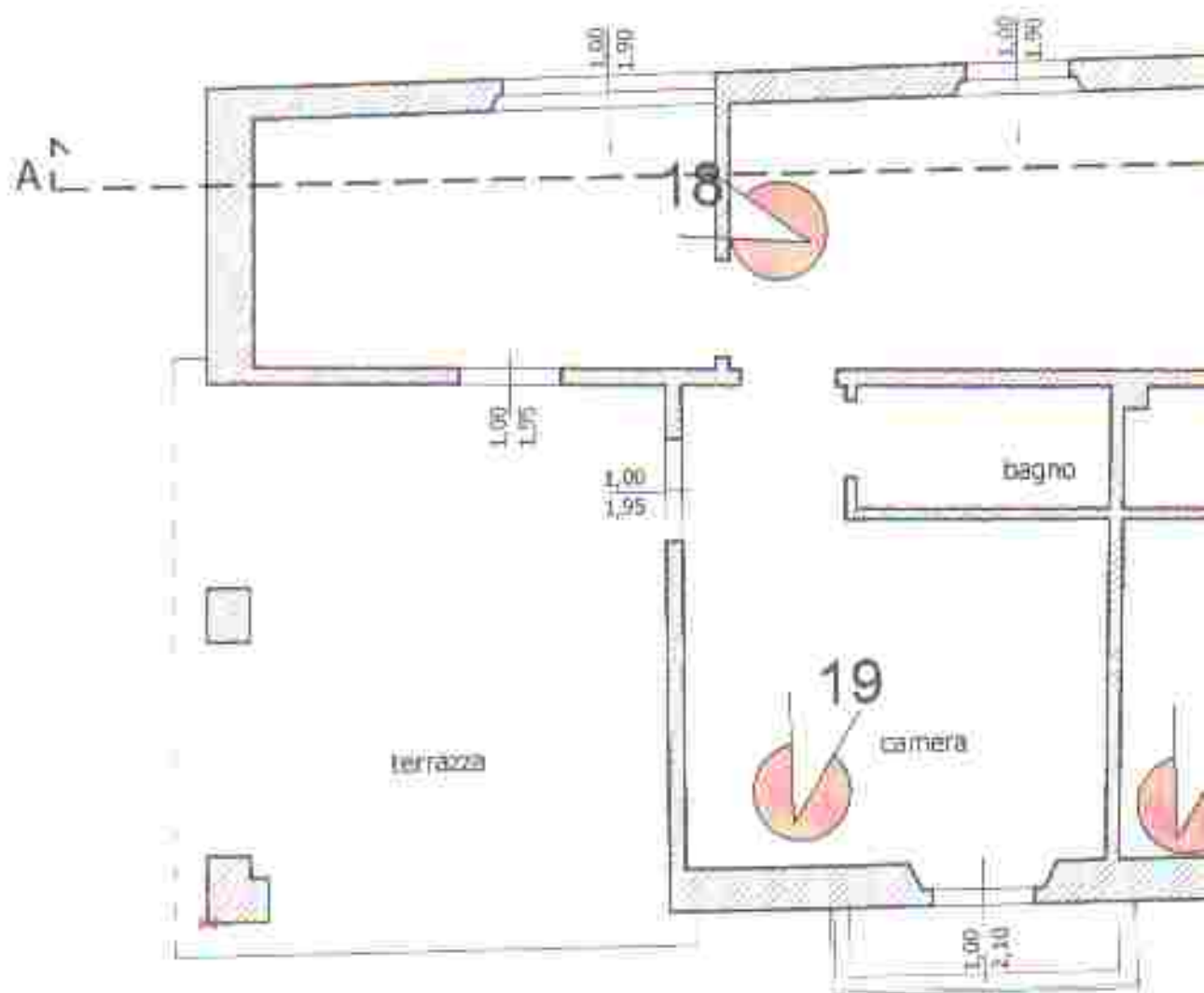
Pianta piano secondo (sottotetto)
